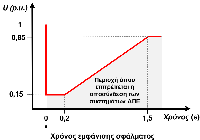
ΣΧΕΔΙΑΓΡΑΜΜΑ 1: Χαρακτηριστική καμπύλη UVRT
