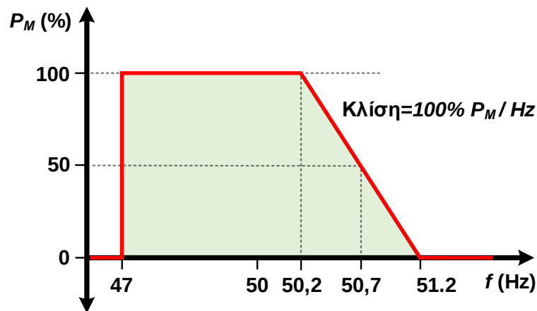
Εικόνα 3: Χαρακτηριστική καμπύλη διακύμανσης/μεταβολής της παραγόμενης ενεργού ισχύος ανάλογα με τη συχνότητα του δικτύου ( P_M : Παραγόμενη ενεργός ισχύς τη στιγμή που η ενεργός ισχύς υπερβαίνει τα 50,2 Hz).
