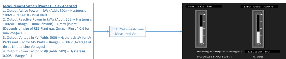
Εικόνα 4.5: Μετρήσεις παραγωγής στο σημείο σύνδεσης του Συστήματος Παραγωγής Ηλεκτρισμού από ΑΠΕ
