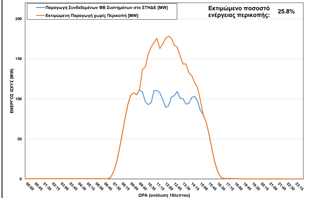
ΦΒ Παραγωγή στο ΣΤΗΔΕ στις 05/01/2024 (ώρα περικοπής: 10:00 - 15:00)
