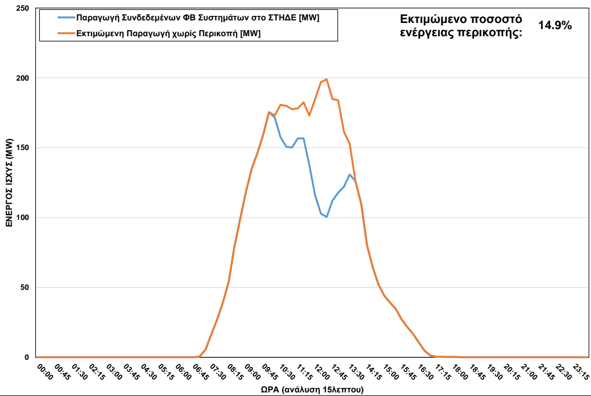
ΦΒ Παραγωγή στο ΣΤΗΔΕ στις 19/01/2024 (ώρα περικοπής: 10:15 - 13:30)
