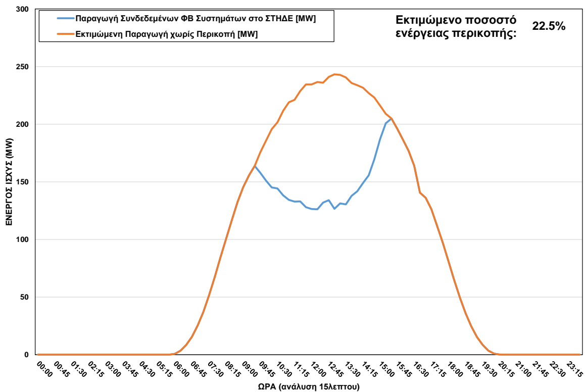
ΦΒ Παραγωγή στο ΣΤΗΔΕ στις 14/07/2024 (ώρα περικοπής: 09:30 - 15:15)
