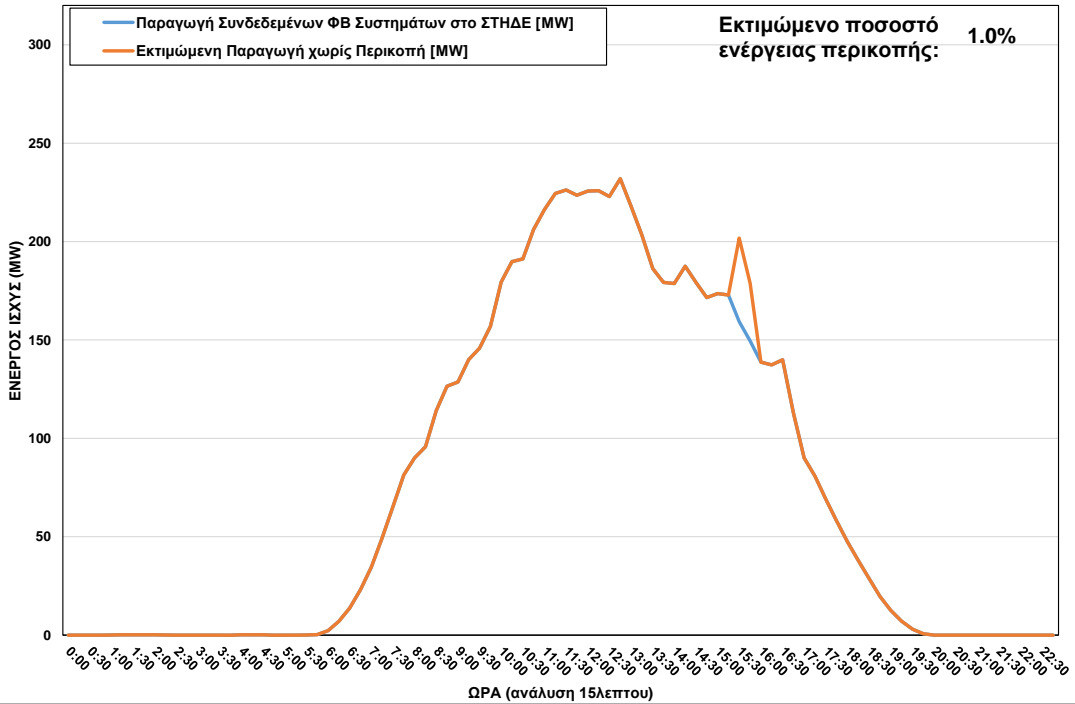
ΦΒ Παραγωγή στο ΣΤΗΔΕ στις 22/05/2024 (ώρα περικοπής: 15:30 - 15:45)
