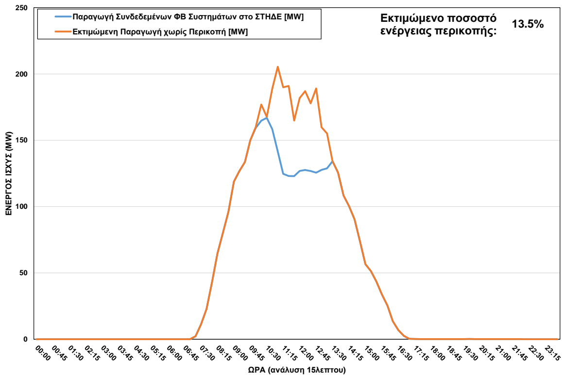
ΦΒ Παραγωγή στο ΣΤΗΔΕ στις 11/01/2024 (ώρα περικοπής: 10:00 - 13:15)
