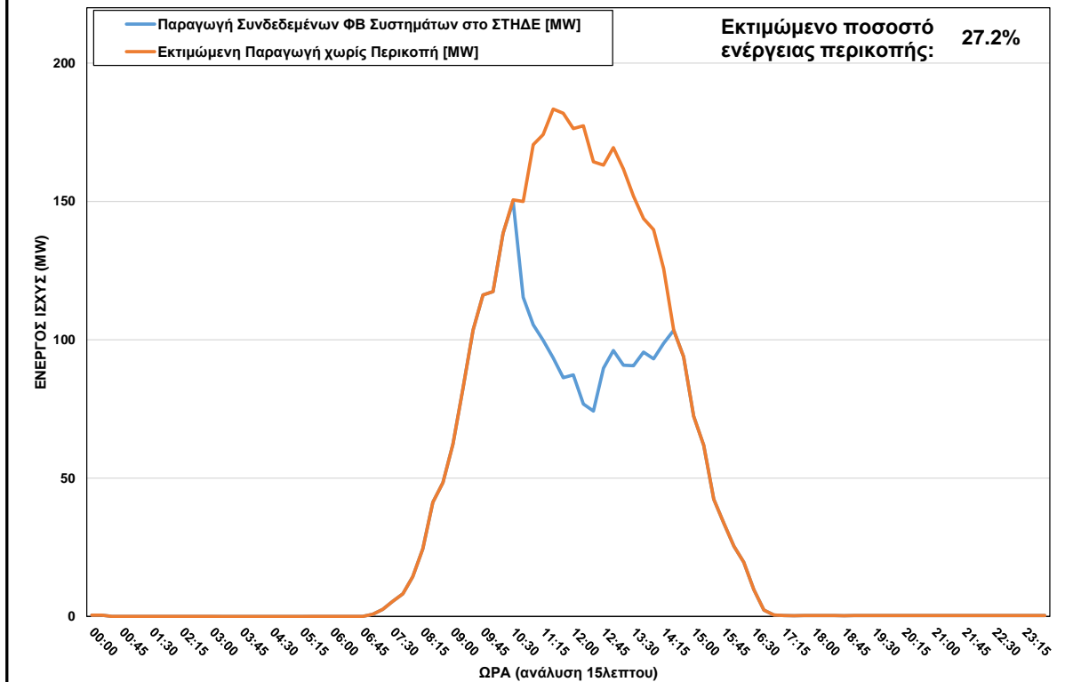
ΦΒ Παραγωγή στο ΣΤΗΔΕ στις 04/01/2024 (ώρα περικοπής: 10:30 - 14:15)
