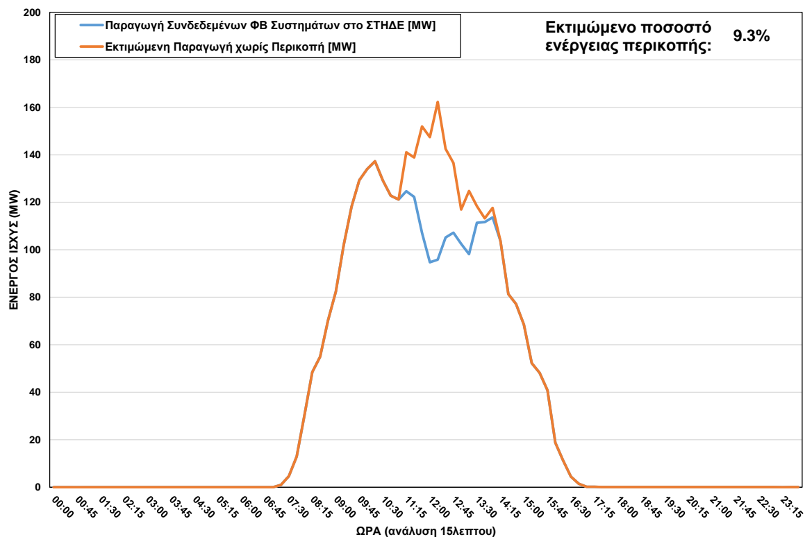
ΦΒ Παραγωγή στο ΣΤΗΔΕ στις 09/01/2024 (ώρα περικοπής: 11:15 - 14:00)
