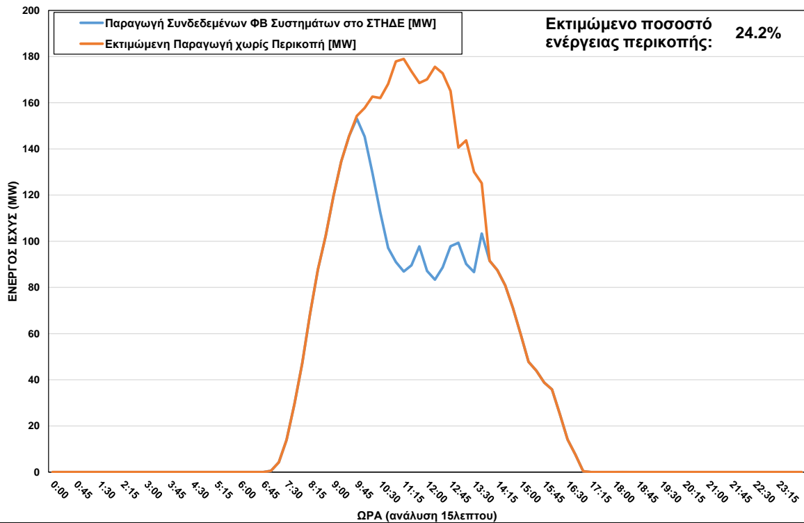
Φ/Β Παραγωγή στο ΣΤΗΔΕ στις 24/01/2024 (ώρα περικοπής: 09:45 - 13:45)
