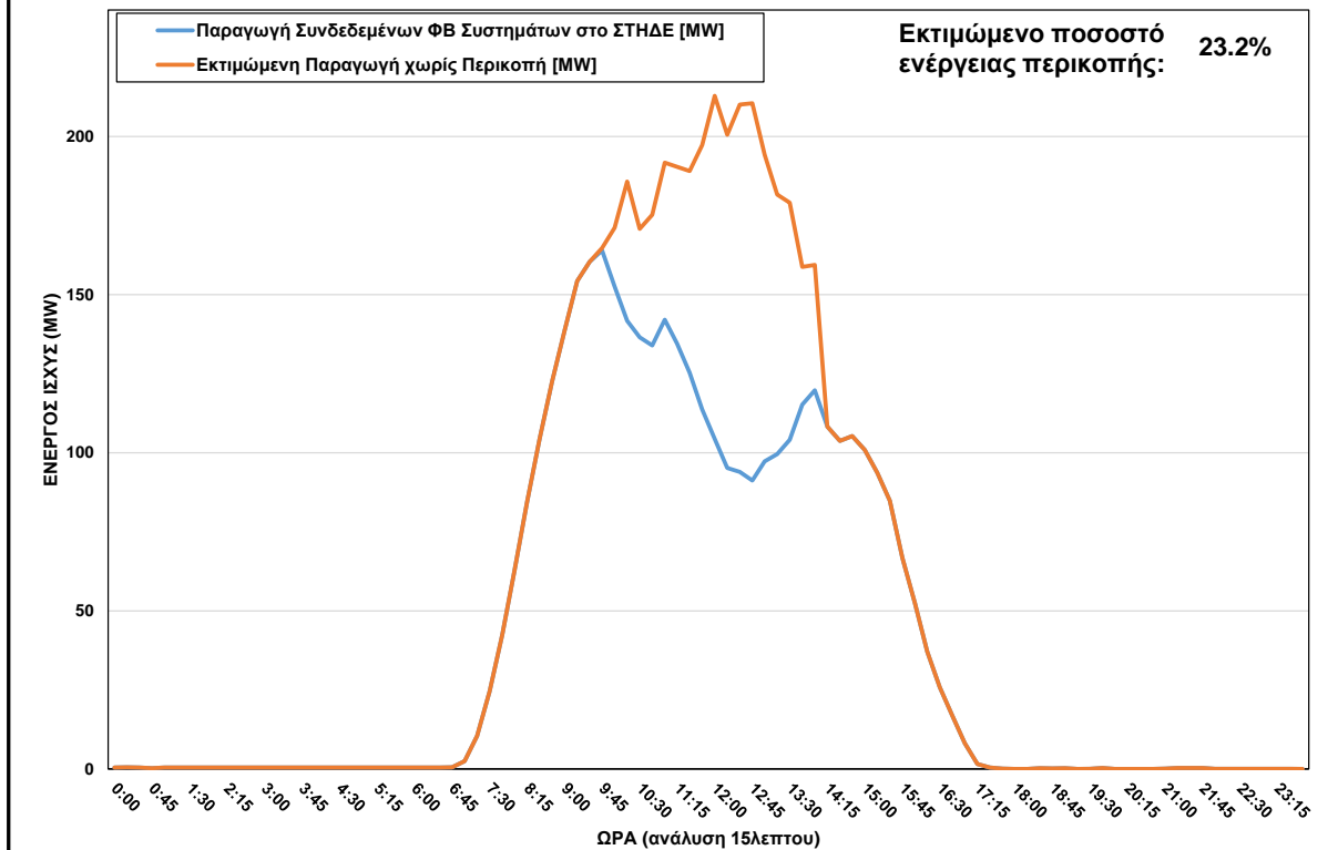
ΦΒ Παραγωγή στο ΣΤΗΔΕ στις 07/02/2024 (ώρα περικοπής: 09:45 - 14:00)
