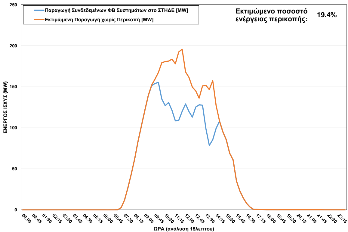
ΦΒ Παραγωγή στο ΣΤΗΔΕ στις 15/01/2024 (ώρα περικοπής: 09:30 - 14:15)
