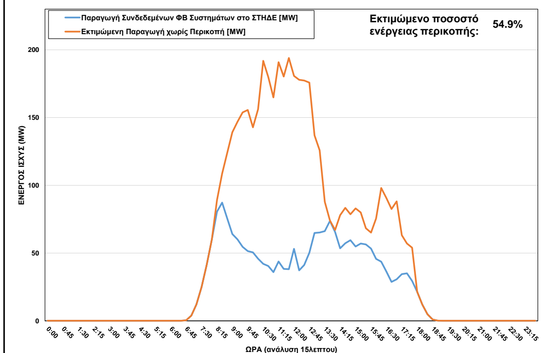
ΦΒ Παραγωγή στο ΣΤΗΔΕ στις 22/09/2024 (ώρα περικοπής: 08:15 - 17:45)
