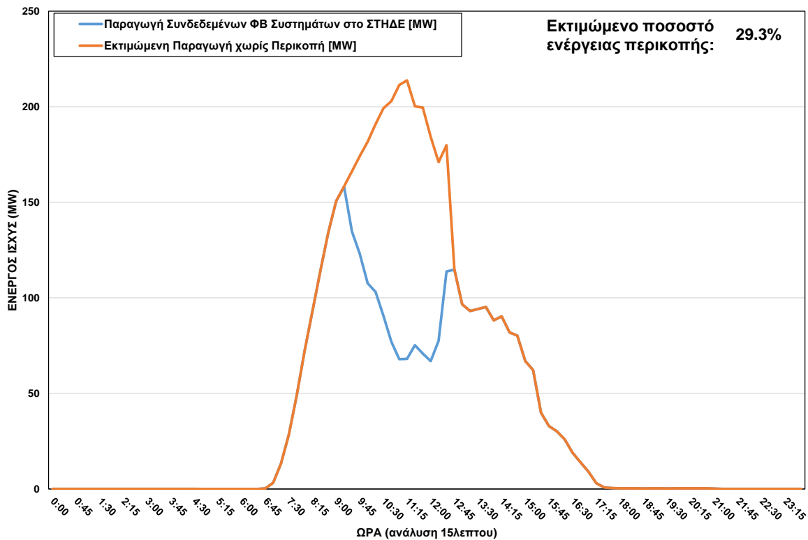
ΦΒ Παραγωγή στο ΣΤΗΔΕ στις 09/02/2024 (ώρα περικοπής: 09:15 - 12:30)
