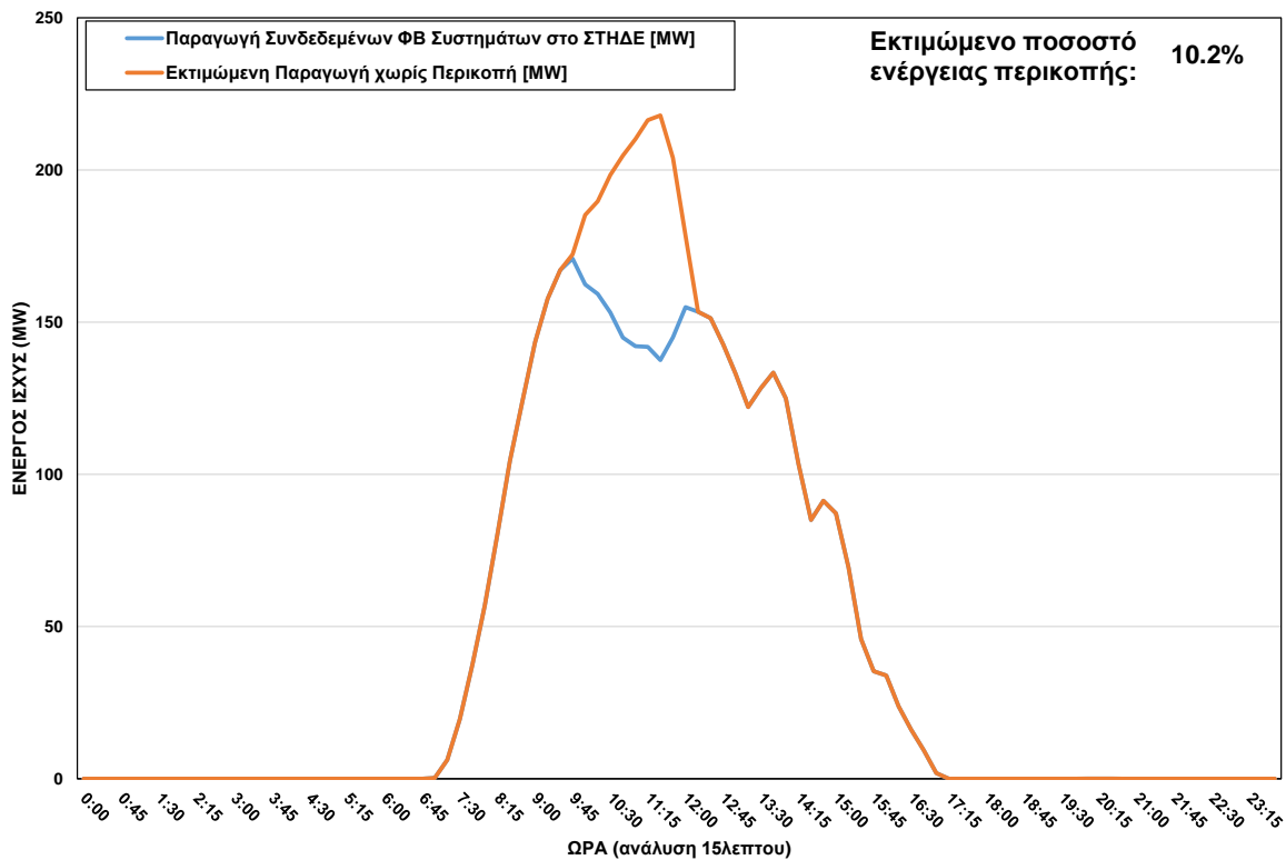
ΦΒ Παραγωγή στο ΣΤΗΔΕ στις 28/01/2024 (ώρα περικοπής: 09:45 - 12:00)
