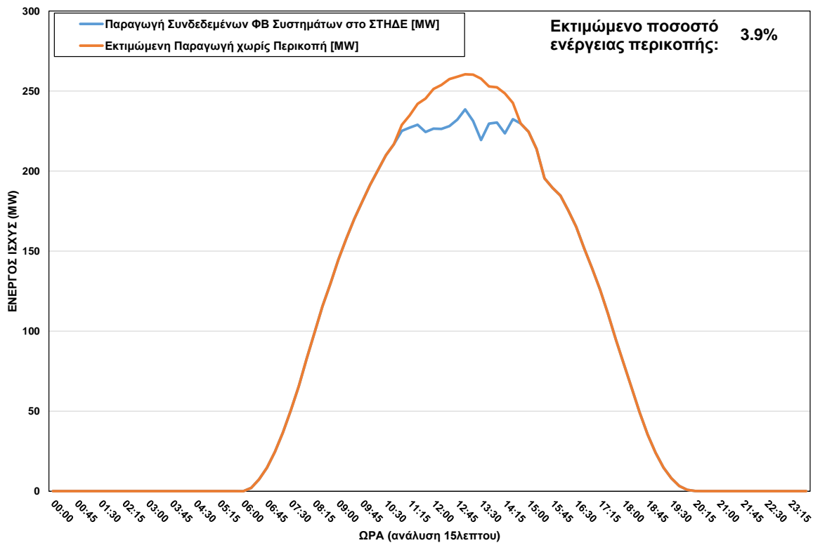
ΦΒ Παραγωγή στο ΣΤΗΔΕ στις 17/07/2024 (ώρα περικοπής: 11:00 - 14:30)
