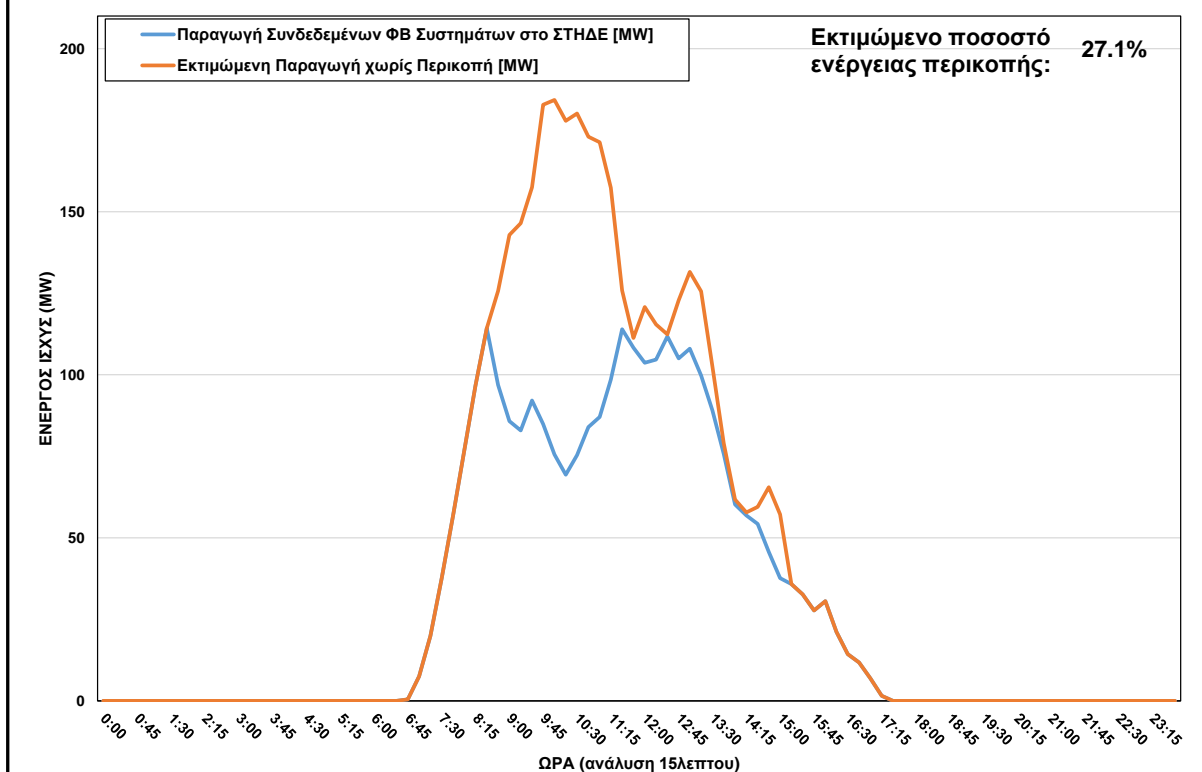
ΦΒ Παραγωγή στο ΣΤΗΔΕ στις 18/02/2024 (ώρα περικοπής: 08:45 - 15:00)
