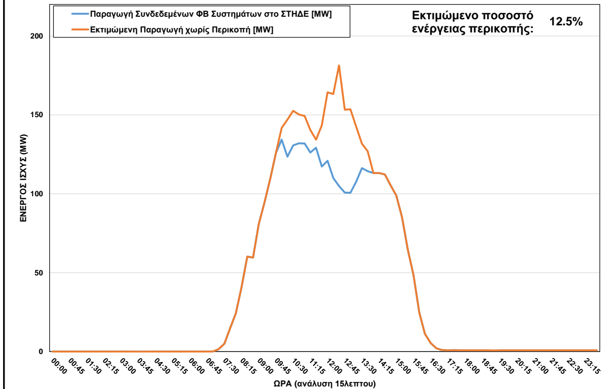
ΦΒ Παραγωγή στο ΣΤΗΔΕ στις 12/01/2024 (ώρα περικοπής: 10:00 - 13:45)
