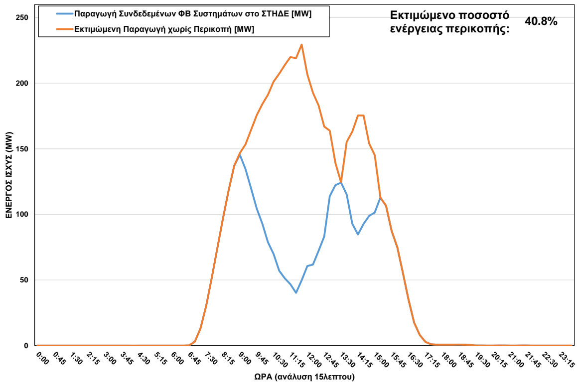
ΦΒ Παραγωγή στο ΣΤΗΔΕ στις 10/02/2024 (ώρα περικοπής: 09:00 - 15:00)
