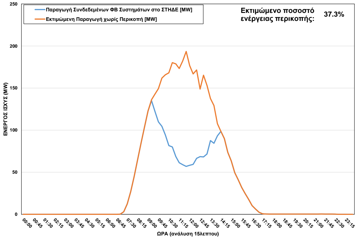
ΦΒ Παραγωγή στο ΣΤΗΔΕ στις 18/01/2024 (ώρα περικοπής: 09:15 - 14:00)
