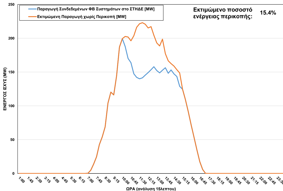
ΦΒ Παραγωγή στο ΣΤΗΔΕ στις 27/01/2024 (ώρα περικοπής: 10:15 - 15:00)
