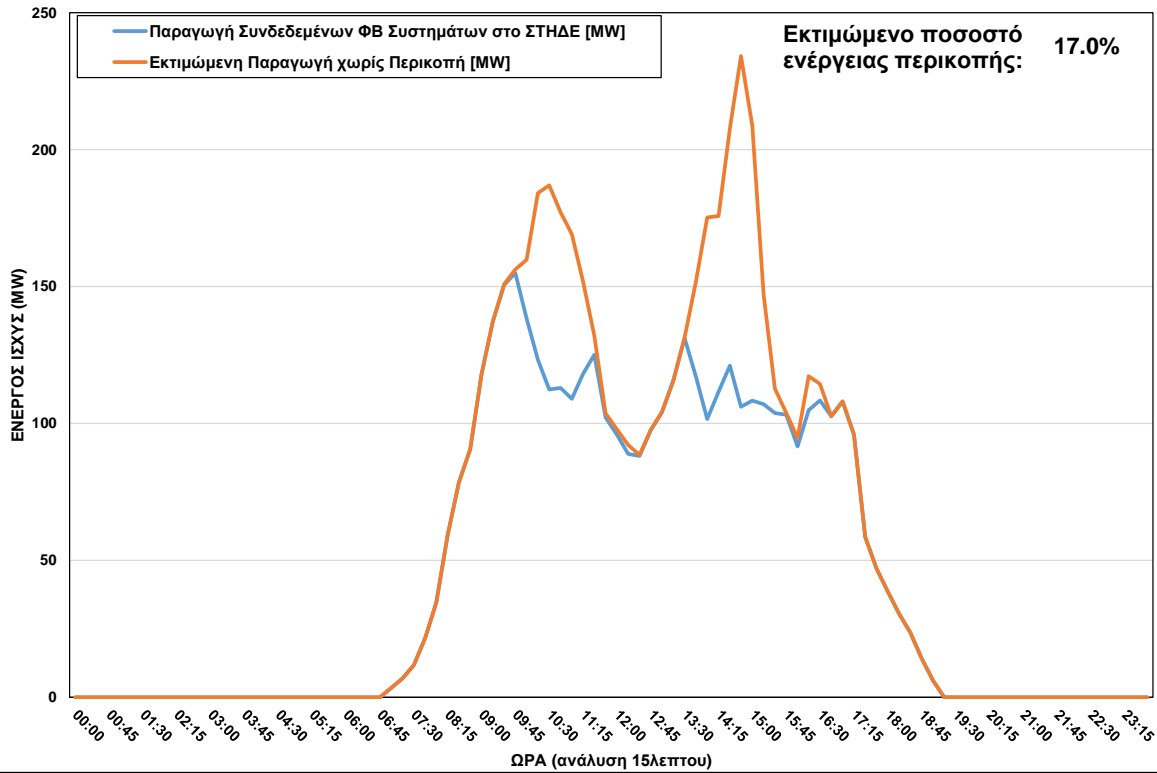
ΦΒ Παραγωγή στο ΣΤΗΔΕ στις 10/04/2024 (ώρα περικοπής: 09:30 - 16:30)
