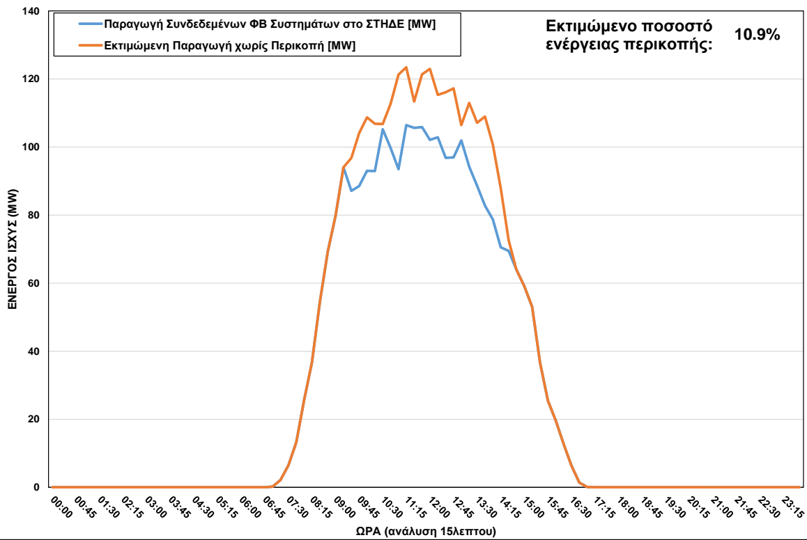
ΦΒ Παραγωγή στο ΣΤΗΔΕ στις 07/01/2024 (ώρα περικοπής: 09:30 - 14:30)
