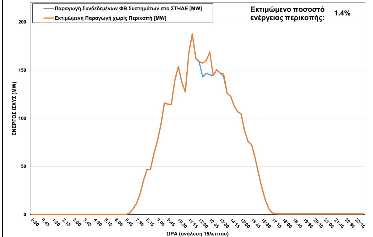
ΦΒ Παραγωγή στο ΣΤΗΔΕ στις 02/02/2024 (ώρα περικοπής: 12:00 - 13:45)
