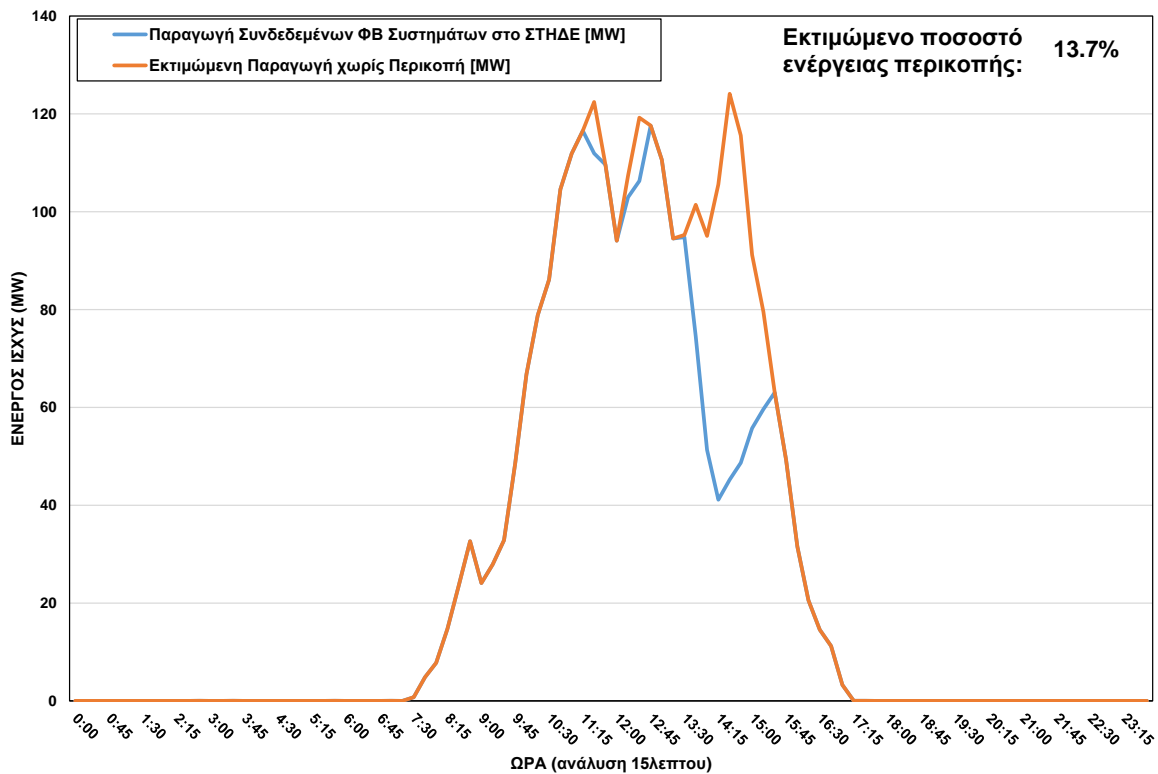
ΦΒ Παραγωγή στο ΣΤΗΔΕ στις 26/01/2024 (ώρα περικοπής: 11:30 - 15:15)
