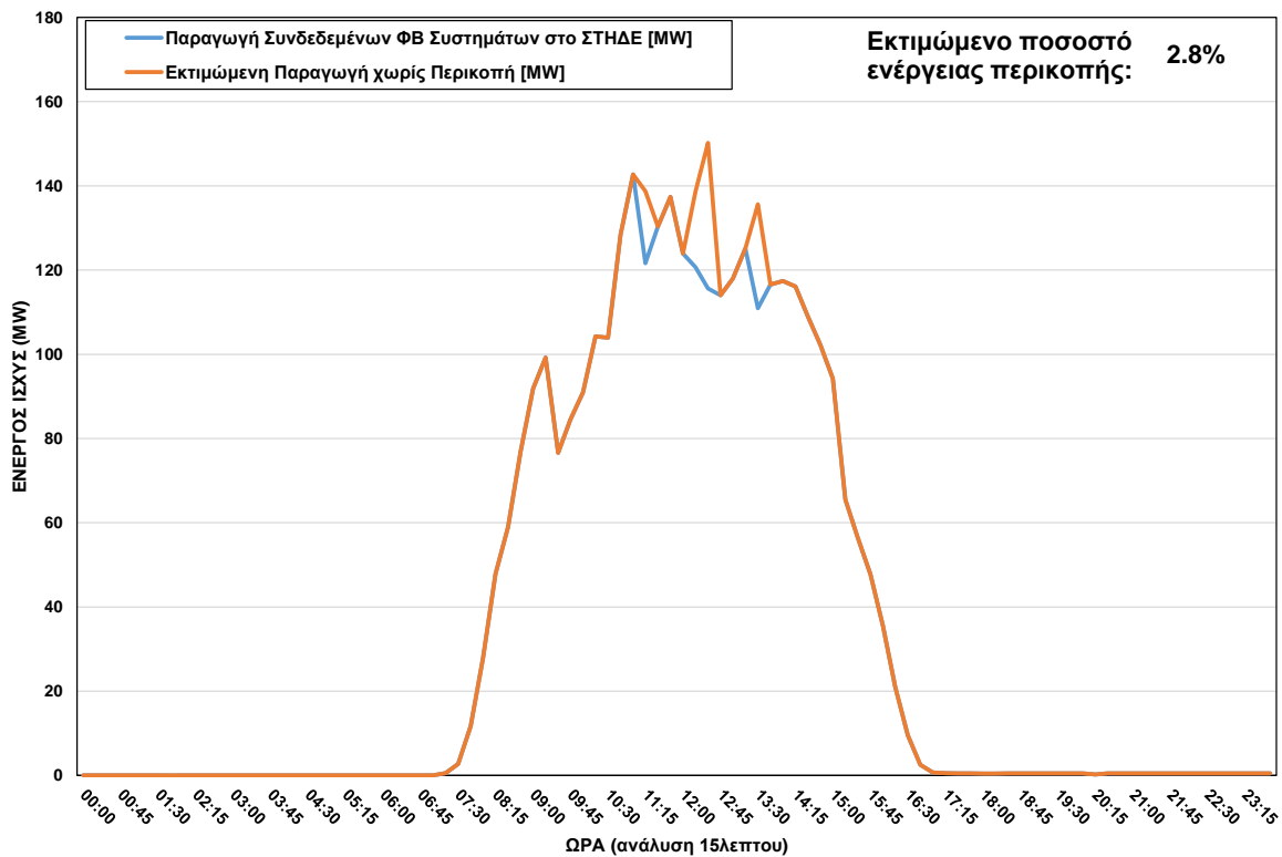
ΦΒ Παραγωγή στο ΣΤΗΔΕ στις 03/01/2024 (ώρα περικοπής: 11:00 - 13:30)
