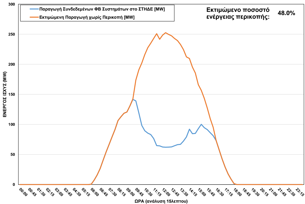
ΦΒ Παραγωγή στο ΣΤΗΔΕ στις 29/03/2024 (ώρα περικοπής: 09:30 - 16:15)
