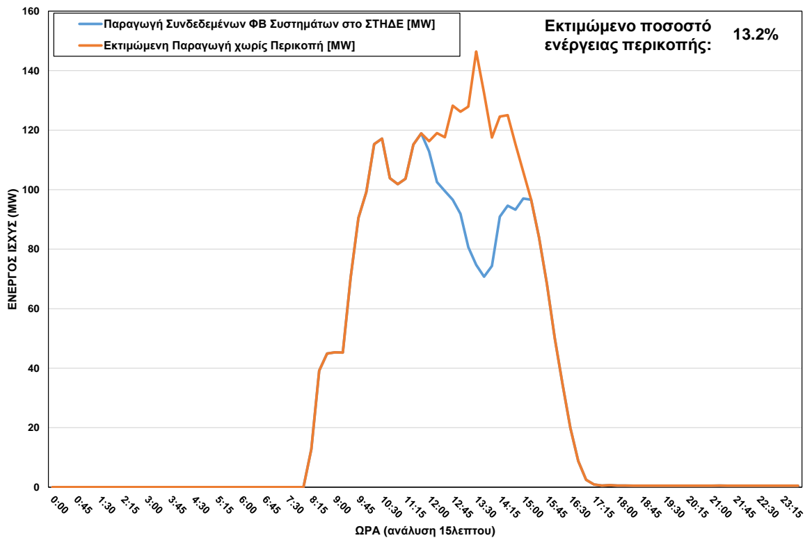
ΦΒ Παραγωγή στο ΣΤΗΔΕ στις 23/01/2024 (ώρα περικοπής: 12:00 - 15:00)
