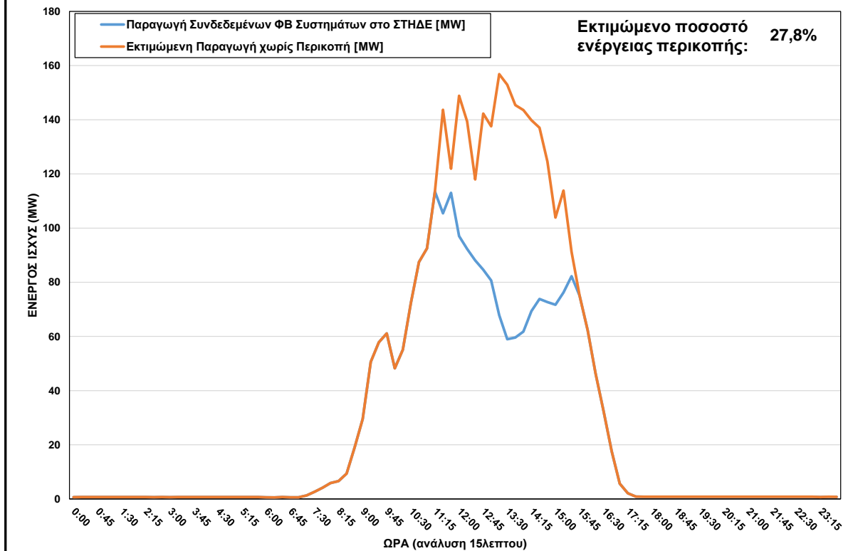
ΦΒ Παραγωγή στο ΣΤΗΔΕ στις 31/01/2024 (ώρα περικοπής: 11:30 - 15:30)
