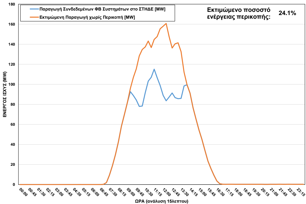
ΦΒ Παραγωγή στο ΣΤΗΔΕ στις 01/01/2024 (ώρα περικοπής: 09:15 - 13:45)
