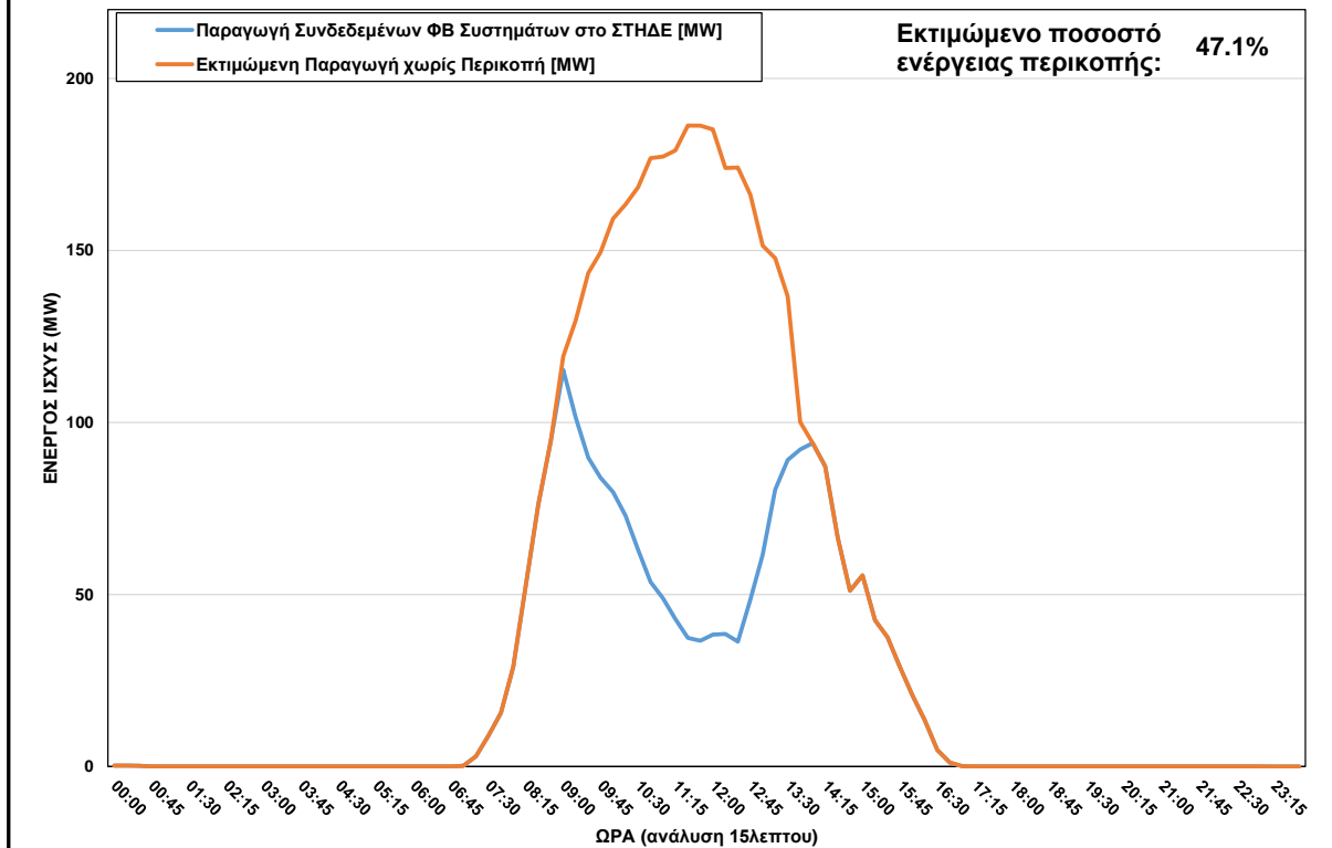
ΦΒ Παραγωγή στο ΣΤΗΔΕ στις 02/01/2024 (ώρα περικοπής: 09:00 - 13:45)
