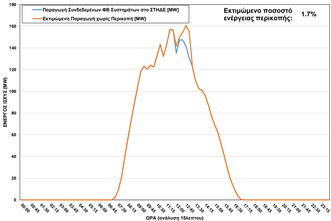
ΦΒ Παραγωγή στο ΣΤΗΔΕ στις 14/01/2024 (ώρα περικοπής: 12:00 - 13:00)
