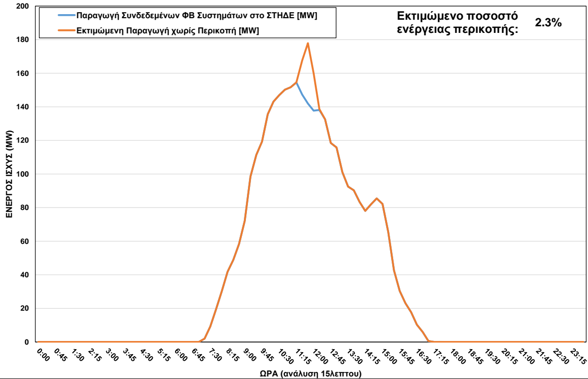
ΦΒ Παραγωγή στο ΣΤΗΔΕ στις 25/01/2024 (ώρα περικοπής: 11:30 - 12:15)
