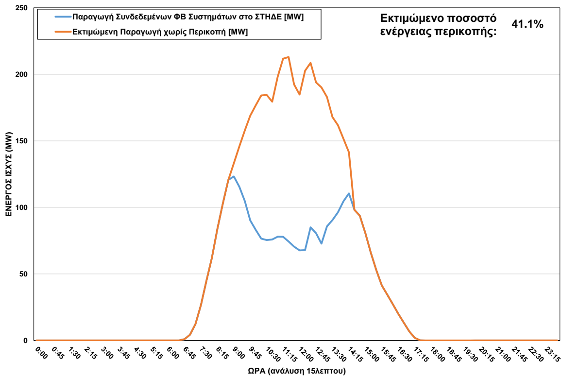
ΦΒ Παραγωγή στο ΣΤΗΔΕ στις 11/02/2024 (ώρα περικοπής: 09:00 - 14:15)
