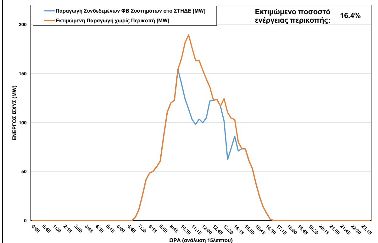
ΦΒ Παραγωγή στο ΣΤΗΔΕ στις 29/01/2024 (ώρα περικοπής: 10:30 - 14:30)
