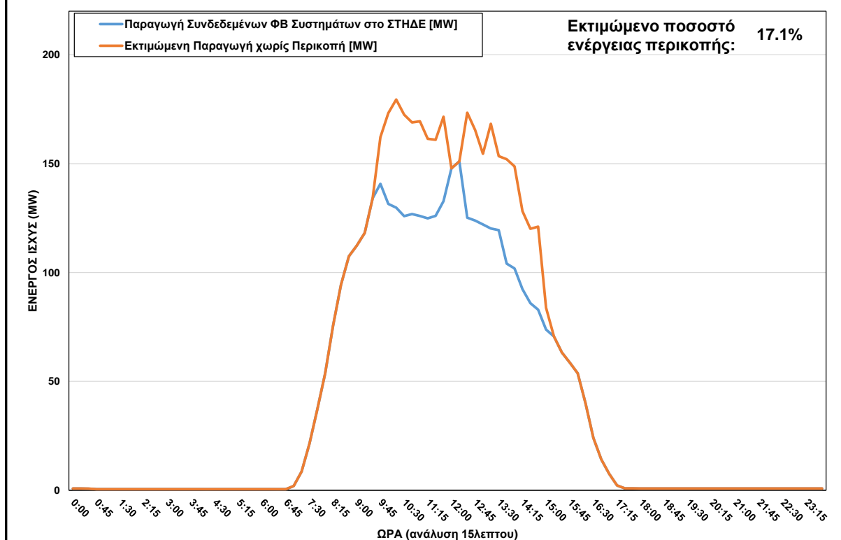
ΦΒ Παραγωγή στο ΣΤΗΔΕ στις 04/02/2024 (ώρα περικοπής: 09:45 - 15:00)
