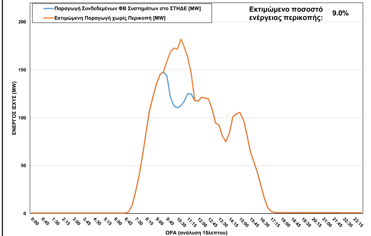
ΦΒ Παραγωγή στο ΣΤΗΔΕ στις 03/02/2024 (ώρα περικοπής: 09:30 - 11:30)
