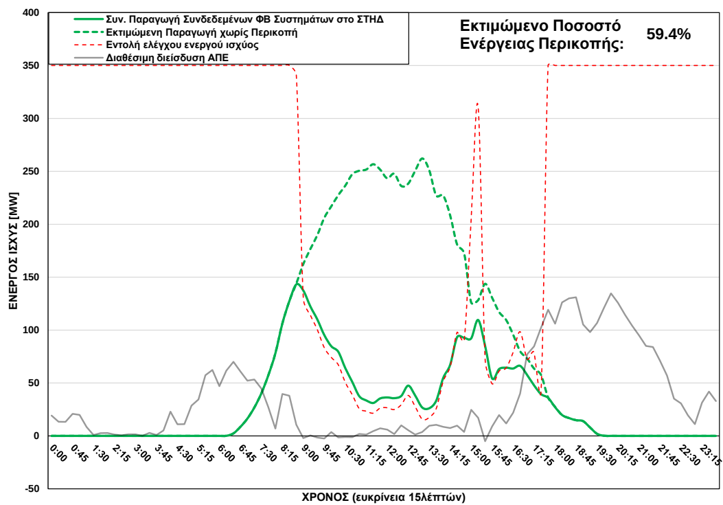
ΦΒ Παραγωγή στο ΣΤΗΔ στις 23/04/2025 (ώρα περικοπής: 08:45 - 17:30)
