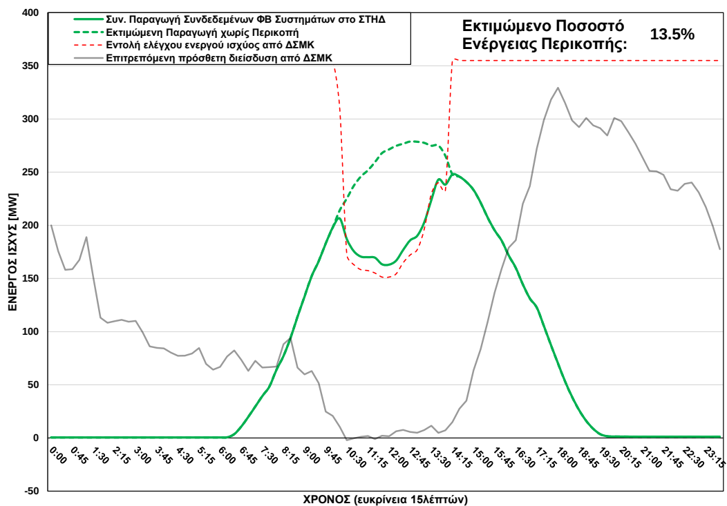
ΦΒ Παραγωγή στο ΣΤΗΔ στις 14/08/2025 (ώρα περικοπής: 10:15 - 14:00)
