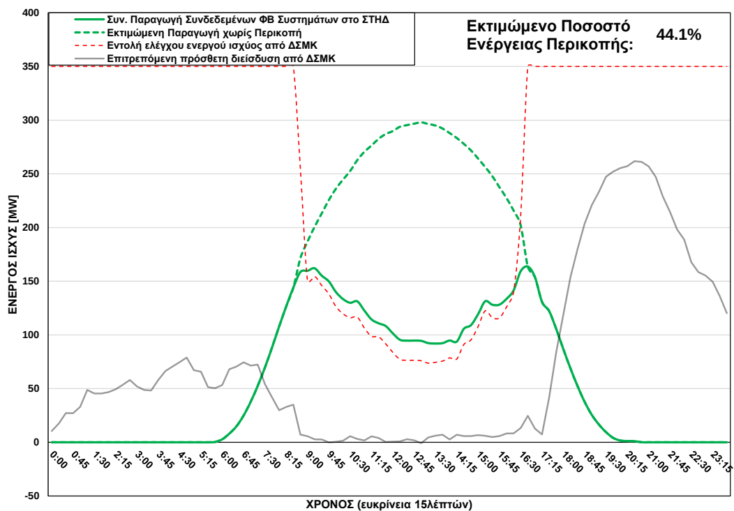
ΦΒ Παραγωγή στο ΣΤΗΔ στις 04/06/2025 (ώρα περικοπής: 08:45 - 16:30)
