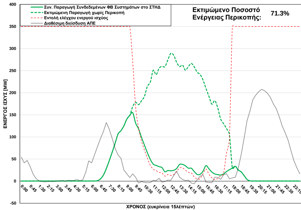
ΦΒ Παραγωγή στο ΣΤΗΔ στις 14/04/2025 (ώρα περικοπής: 09:30 - 17:45)
