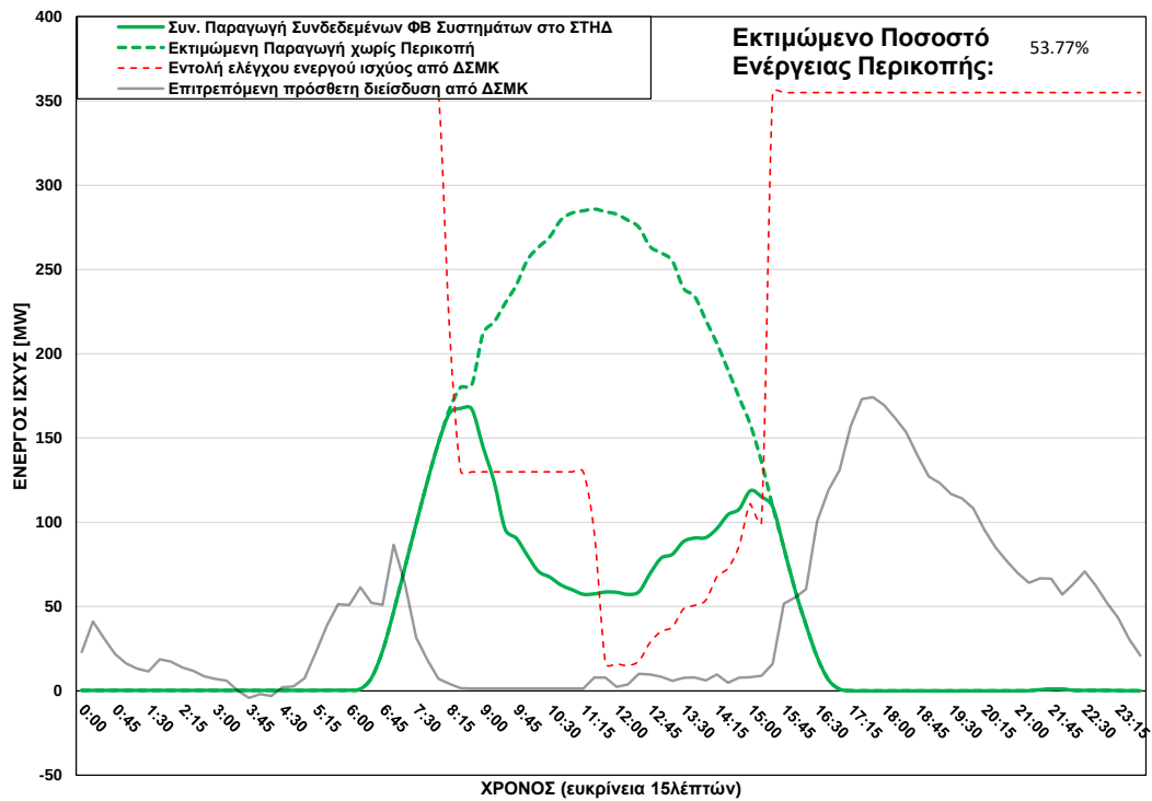
ΦΒ Παραγωγή στο ΣΤΗΔ στις 27/10/2025 (ώρα περικοπής: 08:15 - 15:15)
