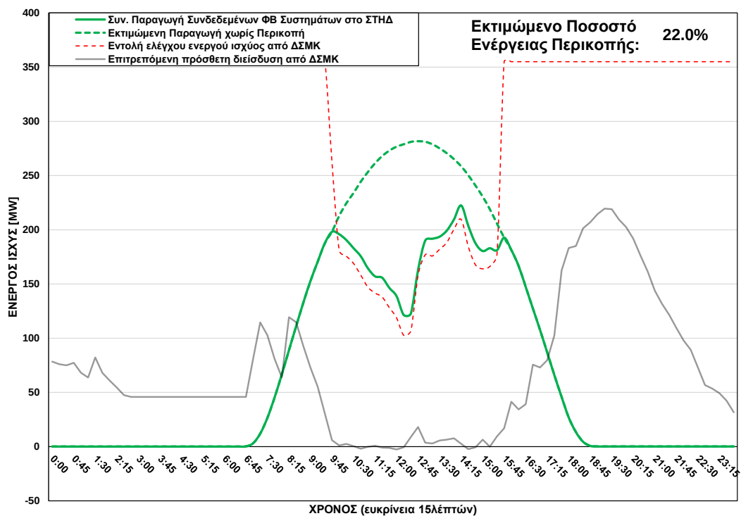
ΦΒ Παραγωγή στο ΣΤΗΔ στις 24/09/2025 (ώρα περικοπής: 09:45 - 15:30)
