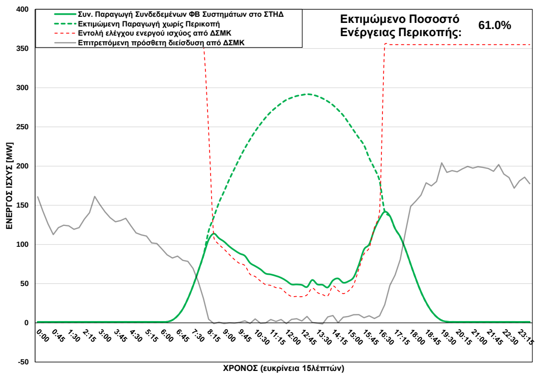
ΦΒ Παραγωγή στο ΣΤΗΔ στις 15/08/2025 (ώρα περικοπής: 08:15 - 16:30)
