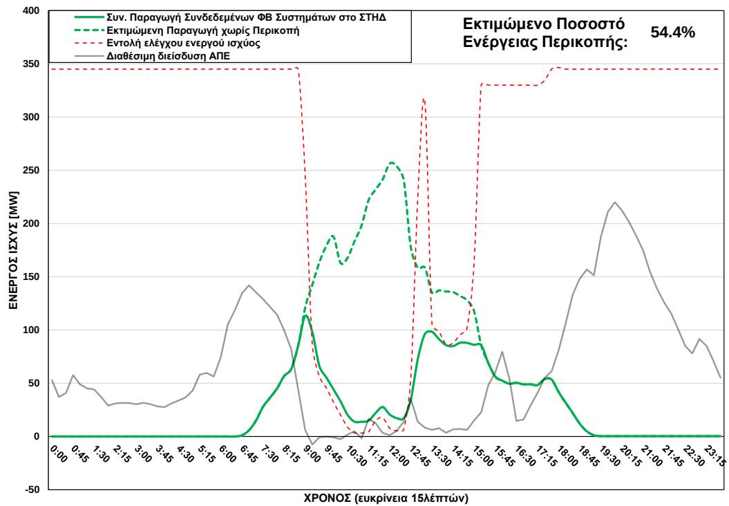
ΦΒ Παραγωγή στο ΣΤΗΔ στις 04/04/2025 (ώρα περικοπής: 09:00 - 15:00)
