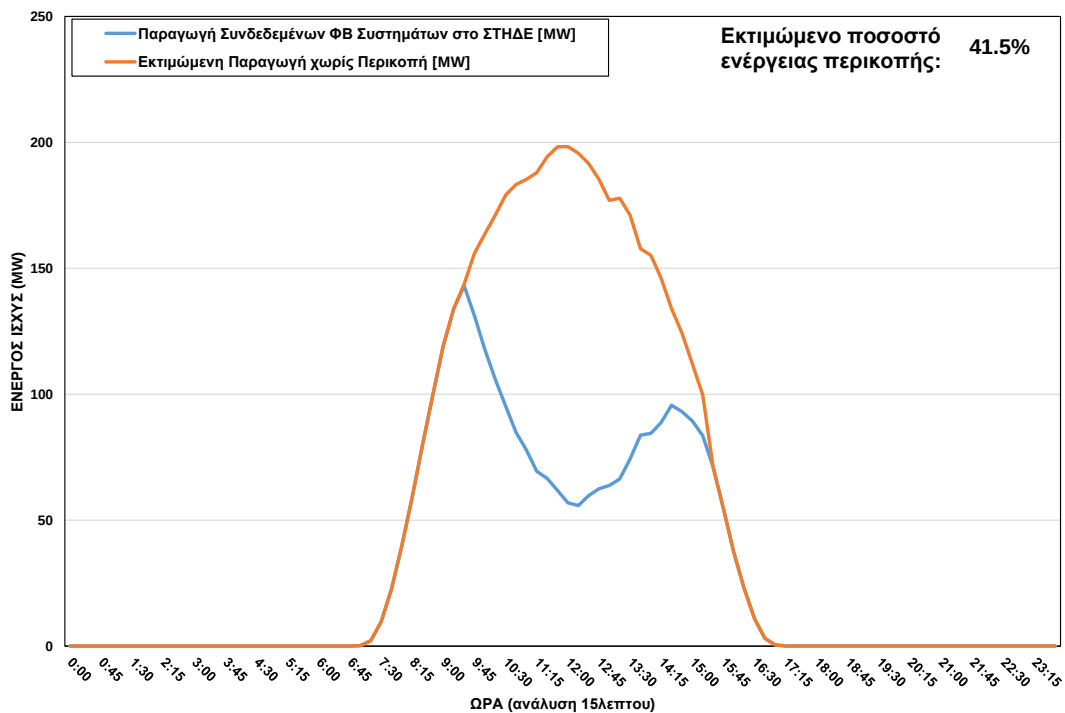
ΦΒ Παραγωγή στο ΣΤΗΔΕ στις 10/01/2025 (ώρα περικοπής: 09:15 - 15:15)
