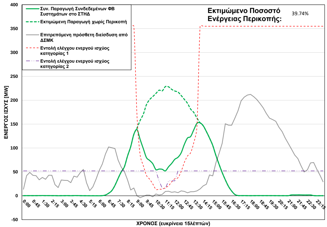
ΦΒ Παραγωγή στο ΣΤΗΔ στις 06/11/2025 (ώρα περικοπής: 09:00 - 13:45)
