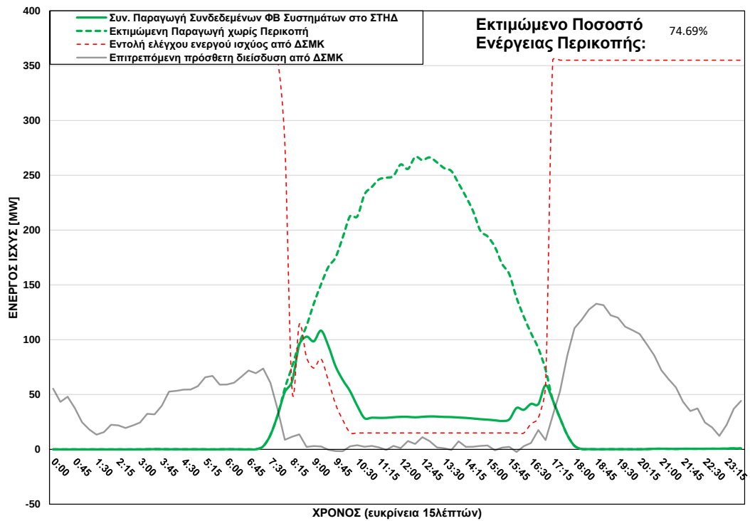
ΦΒ Παραγωγή στο ΣΤΗΔ στις 19/10/2025 (ώρα περικοπής: 08:00 - 17:00)
