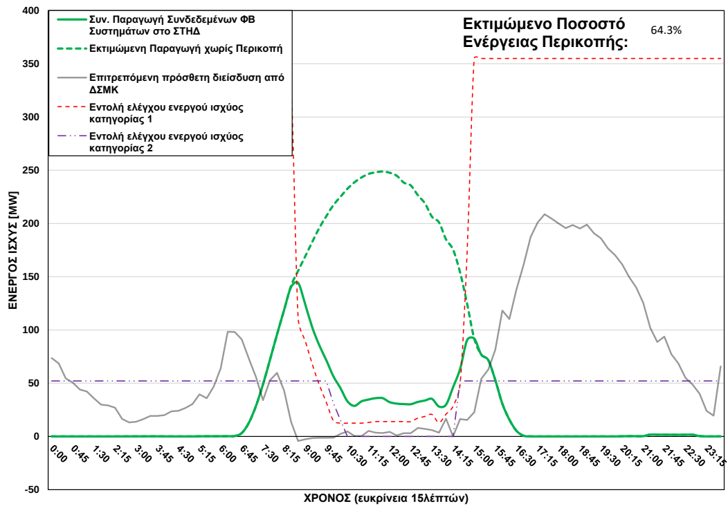
ΦΒ Παραγωγή στο ΣΤΗΔ στις 19/11/2025 (ώρα περικοπής: 08:30 - 14:45)
