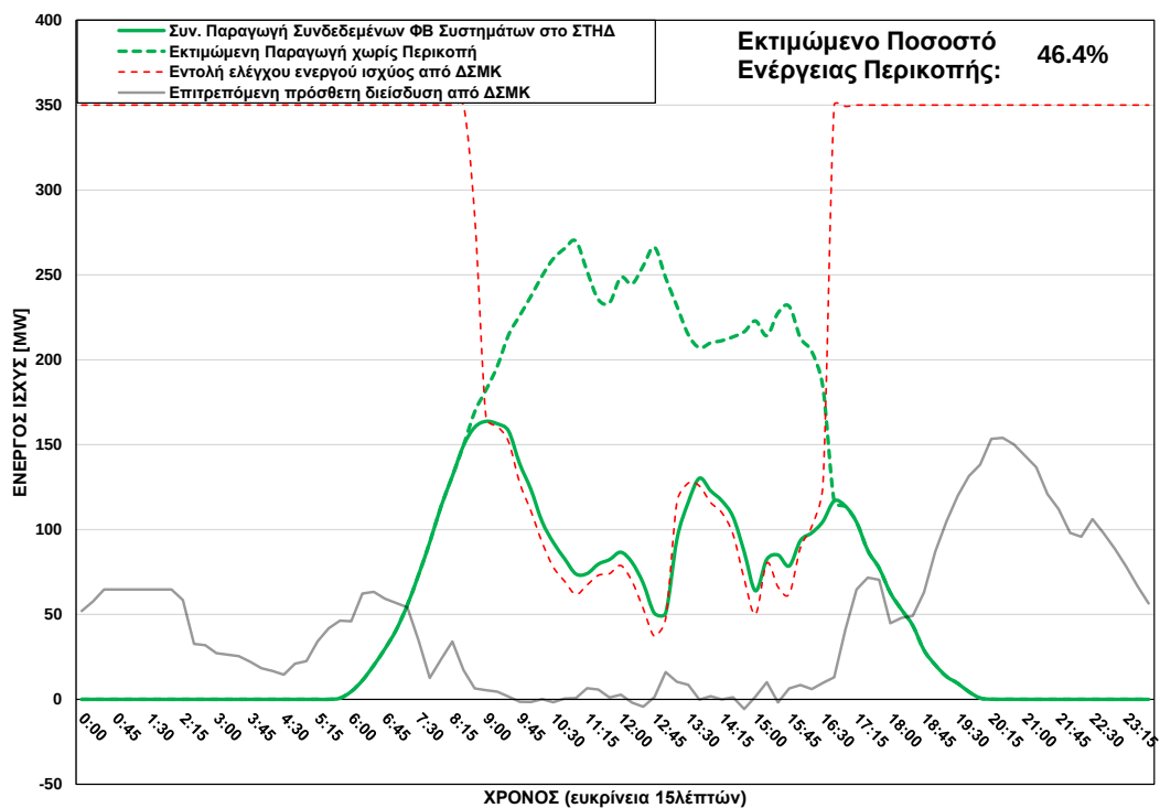
ΦΒ Παραγωγή στο ΣΤΗΔ στις 30/05/2025 (ώρα περικοπής: 08:45 - 16:30)
