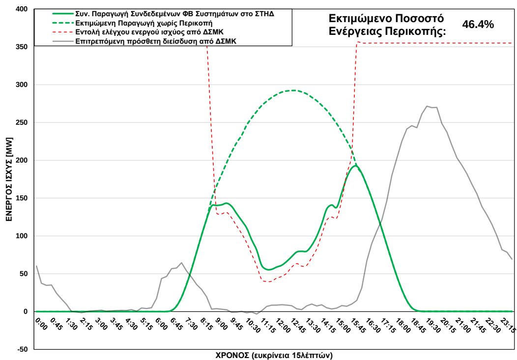
ΦΒ Παραγωγή στο ΣΤΗΔ στις 11/09/2025 (ώρα περικοπής: 08:45 - 15:45)
