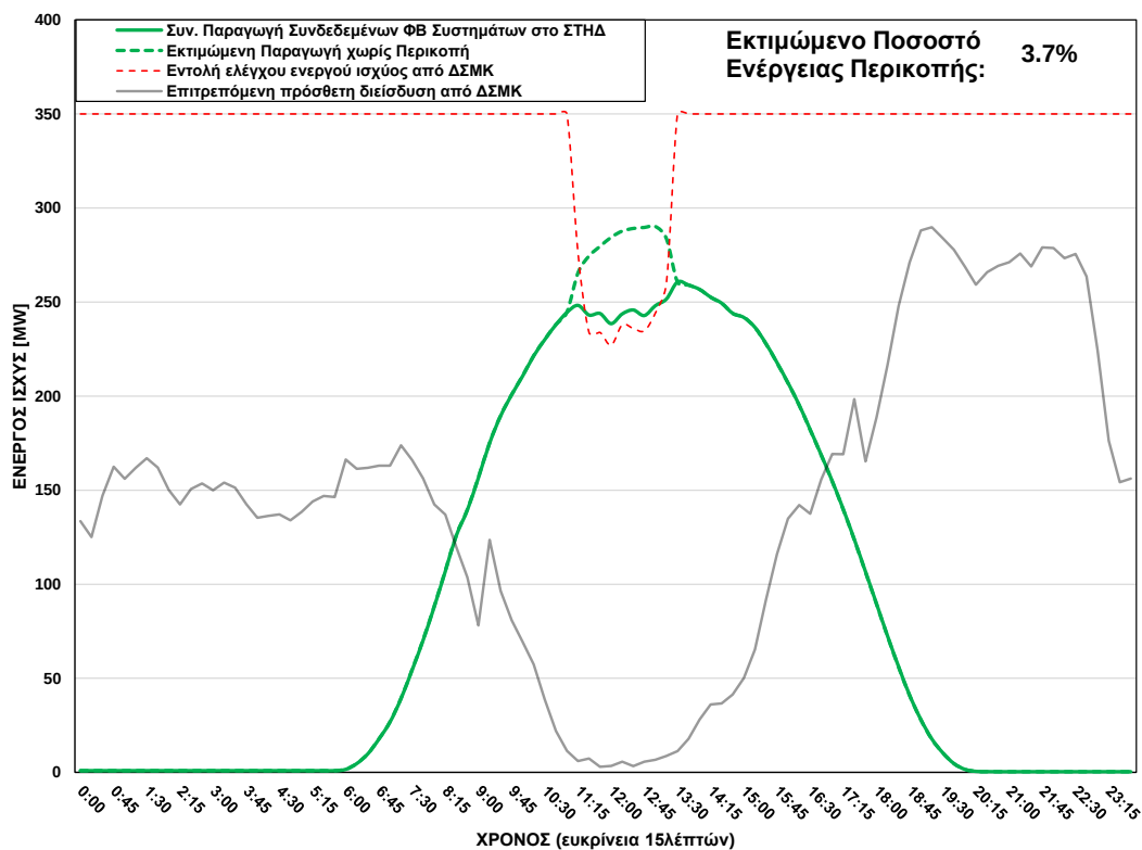
ΦΒ Παραγωγή στο ΣΤΗΔ στις 10/07/2025 (ώρα περικοπής: 11:15 - 13:15)
