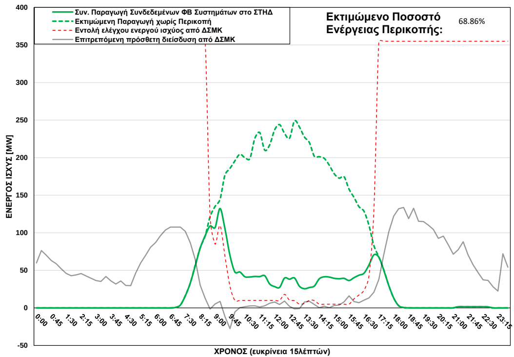
ΦΒ Παραγωγή στο ΣΤΗΔ στις 09/10/2025 (ώρα περικοπής: 08:45 - 17:00)
