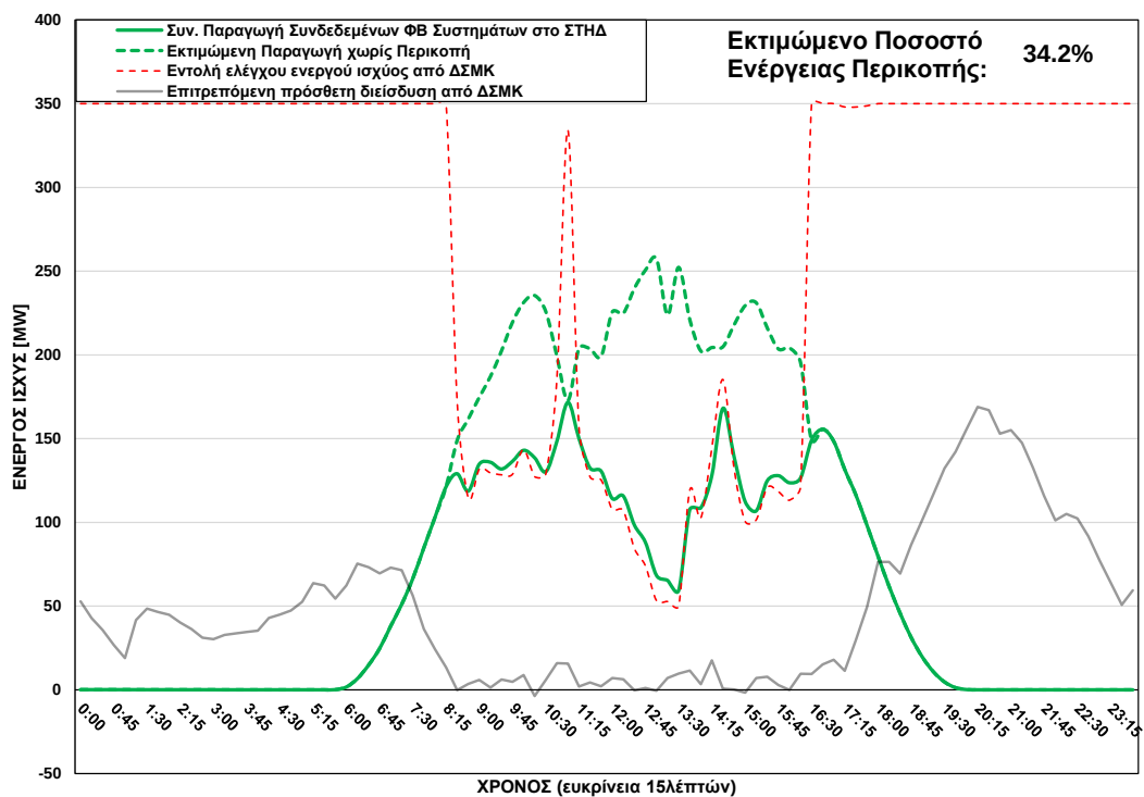
ΦΒ Παραγωγή στο ΣΤΗΔ στις 20/05/2025 (ώρα περικοπής: 08:30 - 16:15)
