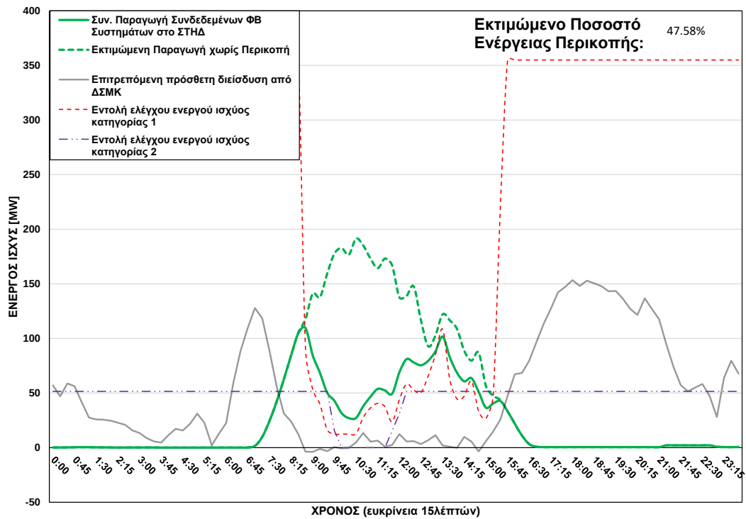
ΦΒ Παραγωγή στο ΣΤΗΔ στις 04/12/2025 (ώρα περικοπής: 08:45 - 15:30)
