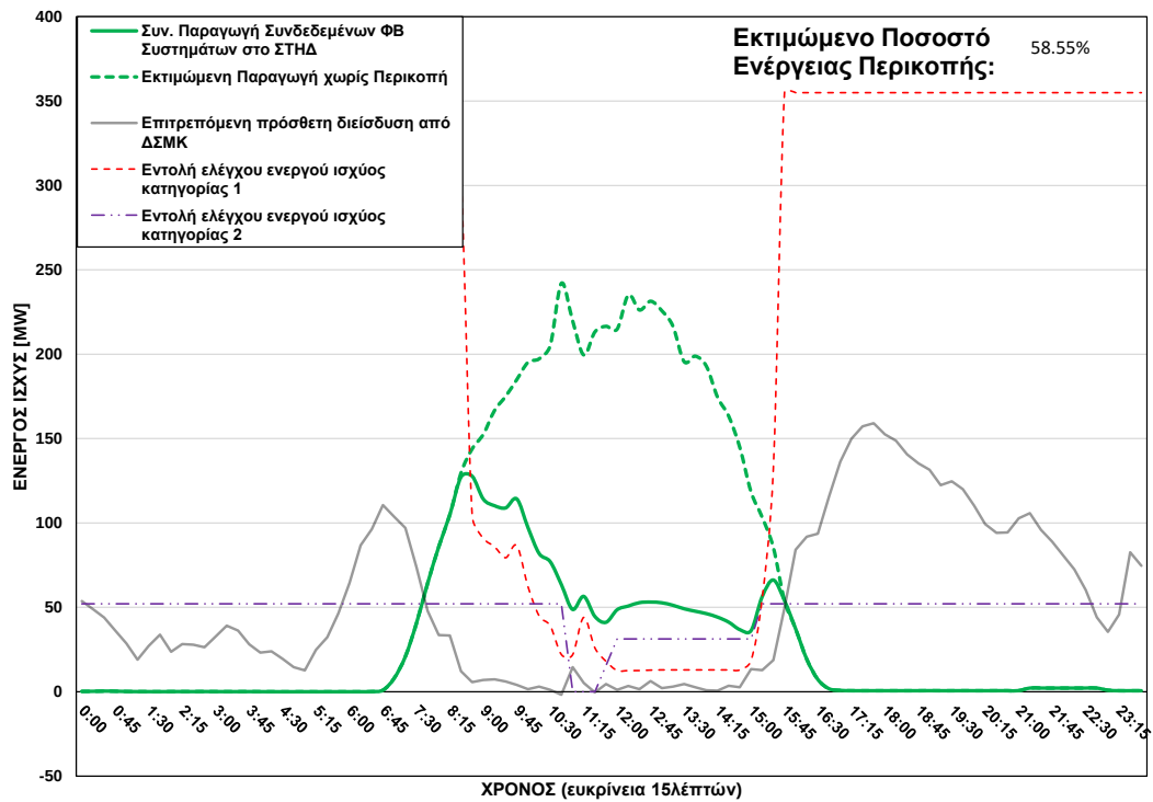
ΦΒ Παραγωγή στο ΣΤΗΔ στις 11/11/2025 (ώρα περικοπής: 08:30 - 15:30)
