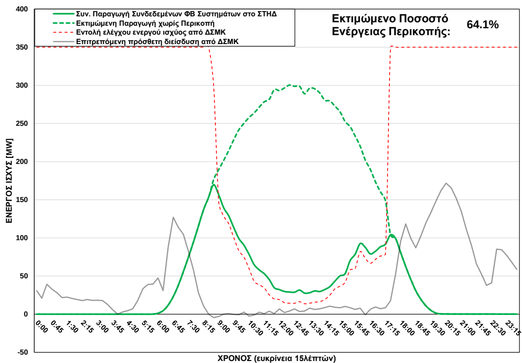
ΦΒ Παραγωγή στο ΣΤΗΔ στις 19/05/2025 (ώρα περικοπής: 08:45 - 17:15)
