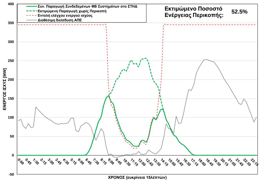
ΦΒ Παραγωγή στο ΣΤΗΔ στις 15/02/2025 (ώρα περικοπής: 09:00 - 14:15)
