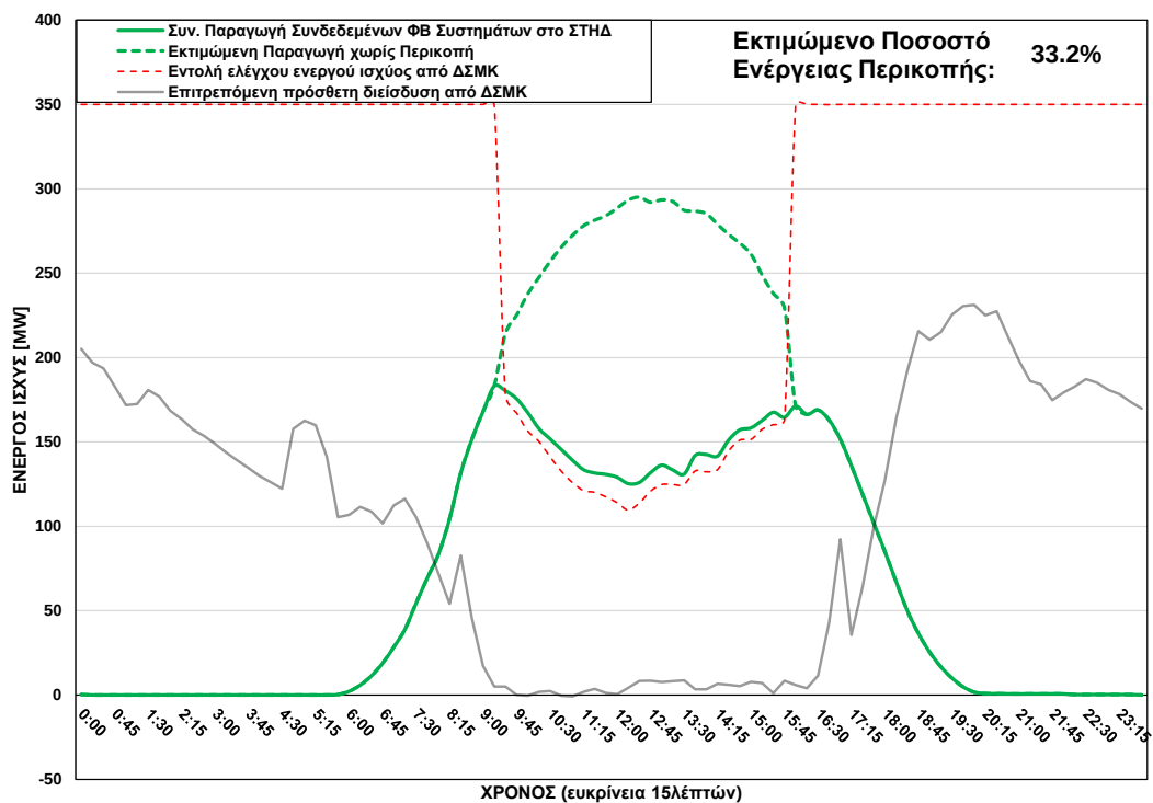
ΦΒ Παραγωγή στο ΣΤΗΔ στις 14/06/2025 (ώρα περικοπής: 09:30 - 15:45)
