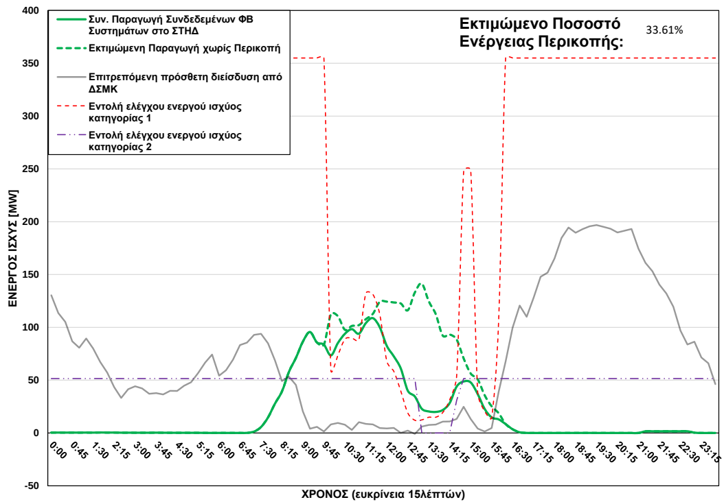
ΦΒ Παραγωγή στο ΣΤΗΔ στις 25/12/2025 (ώρα περικοπής: 10:00 - 16:00)
