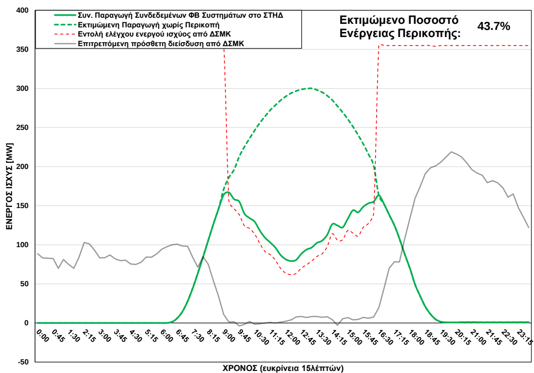
ΦΒ Παραγωγή στο ΣΤΗΔ στις 20/08/2025 (ώρα περικοπής: 09:00 - 16:15)
