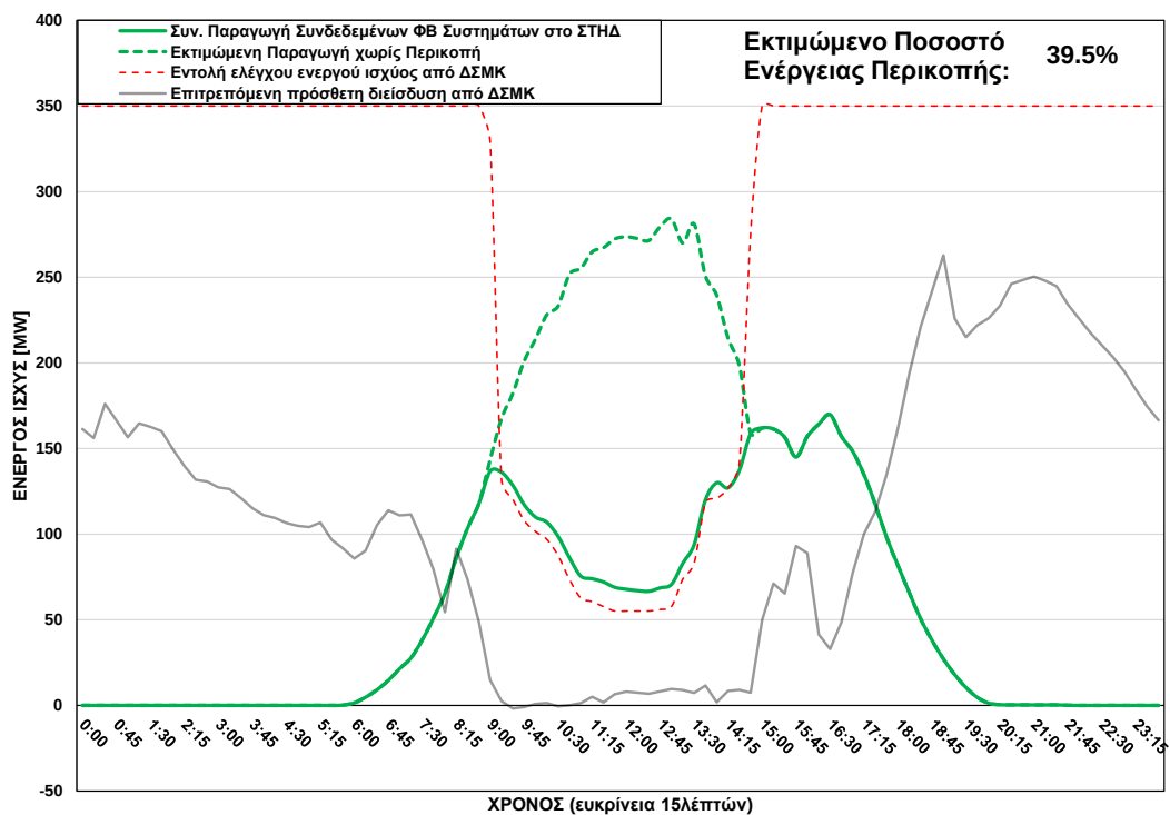
ΦΒ Παραγωγή στο ΣΤΗΔ στις 15/06/2025 (ώρα περικοπής: 09:00 - 14:30)
