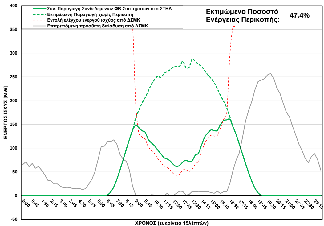
ΦΒ Παραγωγή στο ΣΤΗΔ στις 10/09/2025 (ώρα περικοπής: 09:00 - 16:30)
