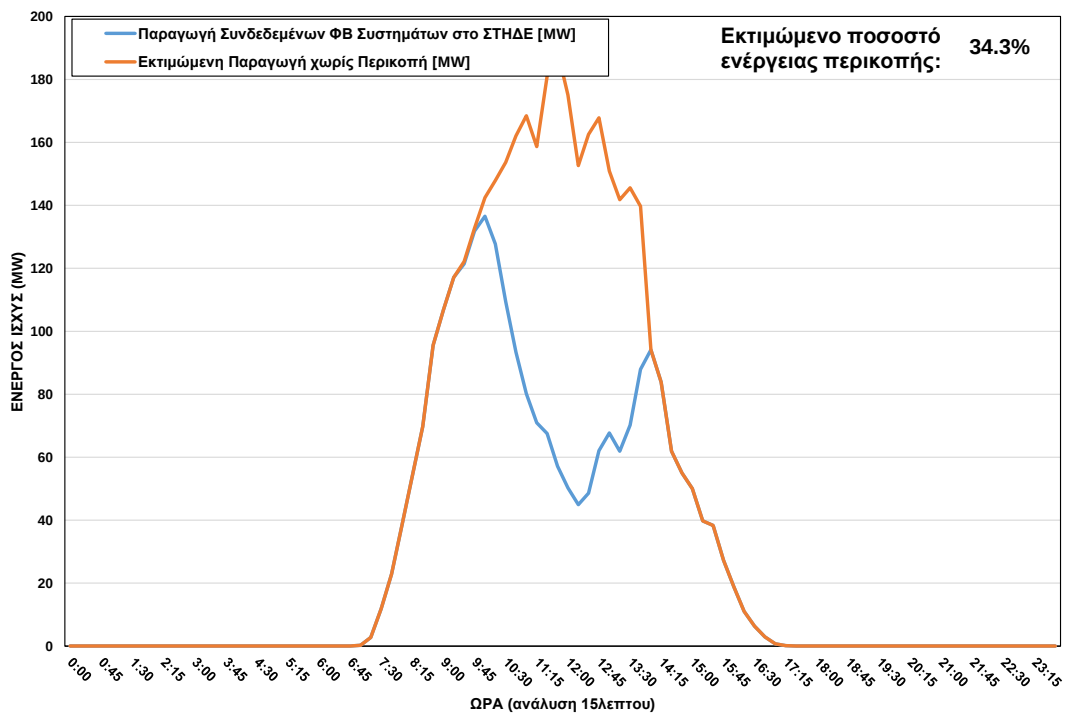
ΦΒ Παραγωγή στο ΣΤΗΔΕ στις 24/01/2025 (ώρα περικοπής: 09:30 - 13:45)
