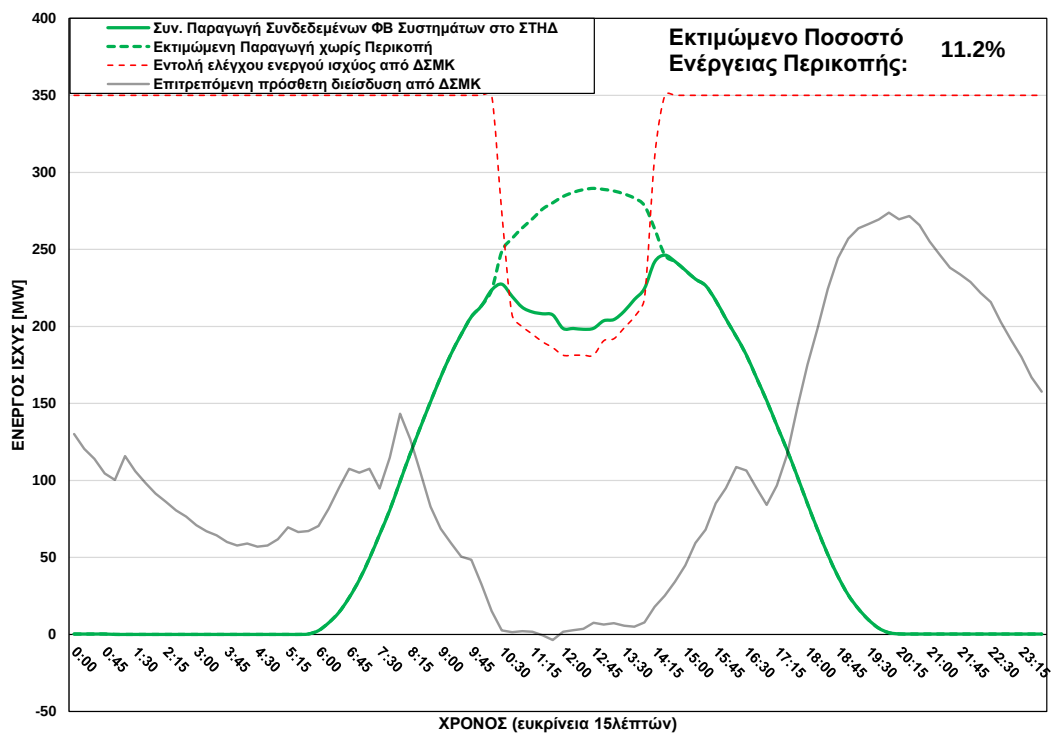
ΦΒ Παραγωγή στο ΣΤΗΔ στις 11/06/2025 (ώρα περικοπής: 10:30 - 14:15)
