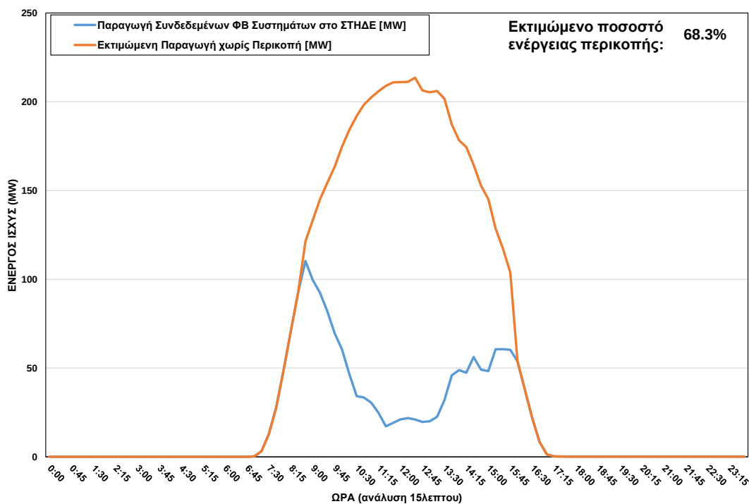
ΦΒ Παραγωγή στο ΣΤΗΔΕ στις 17/01/2025 (ώρα περικοπής: 08:45 - 15:45)
