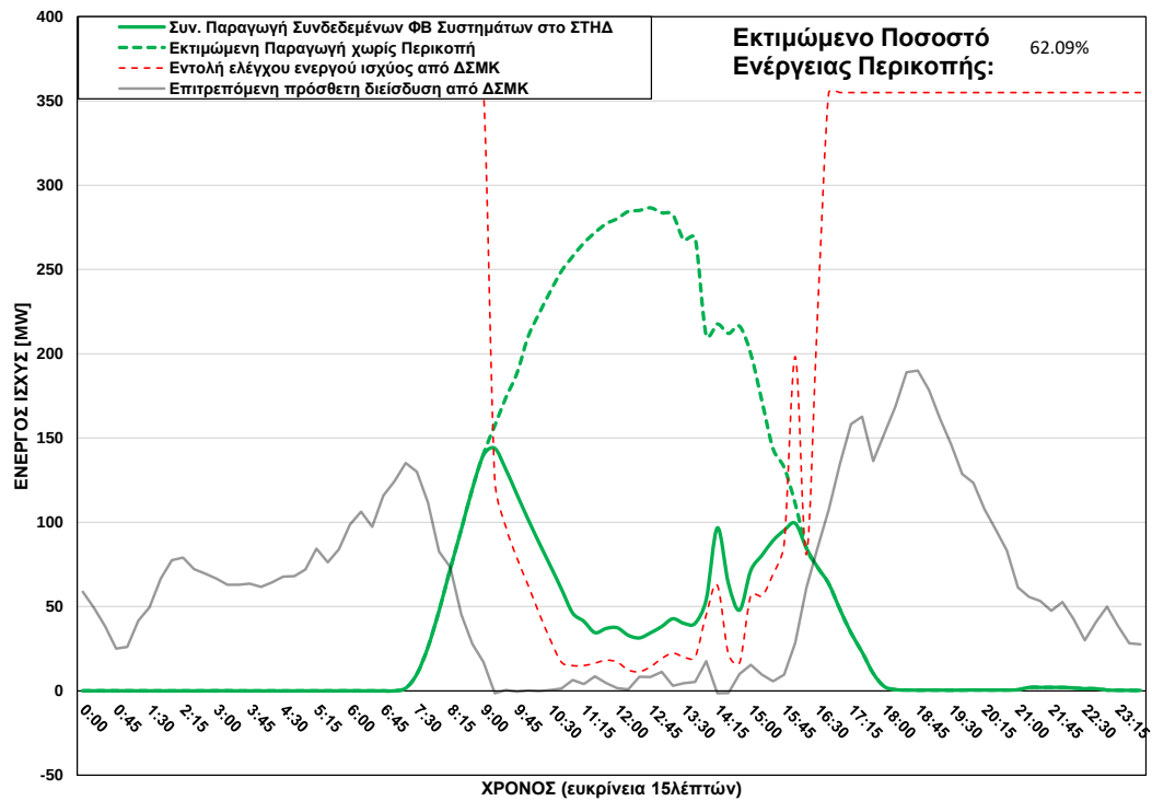
ΦΒ Παραγωγή στο ΣΤΗΔ στις 23/10/2025 (ώρα περικοπής: 09:00 - 16:00)
