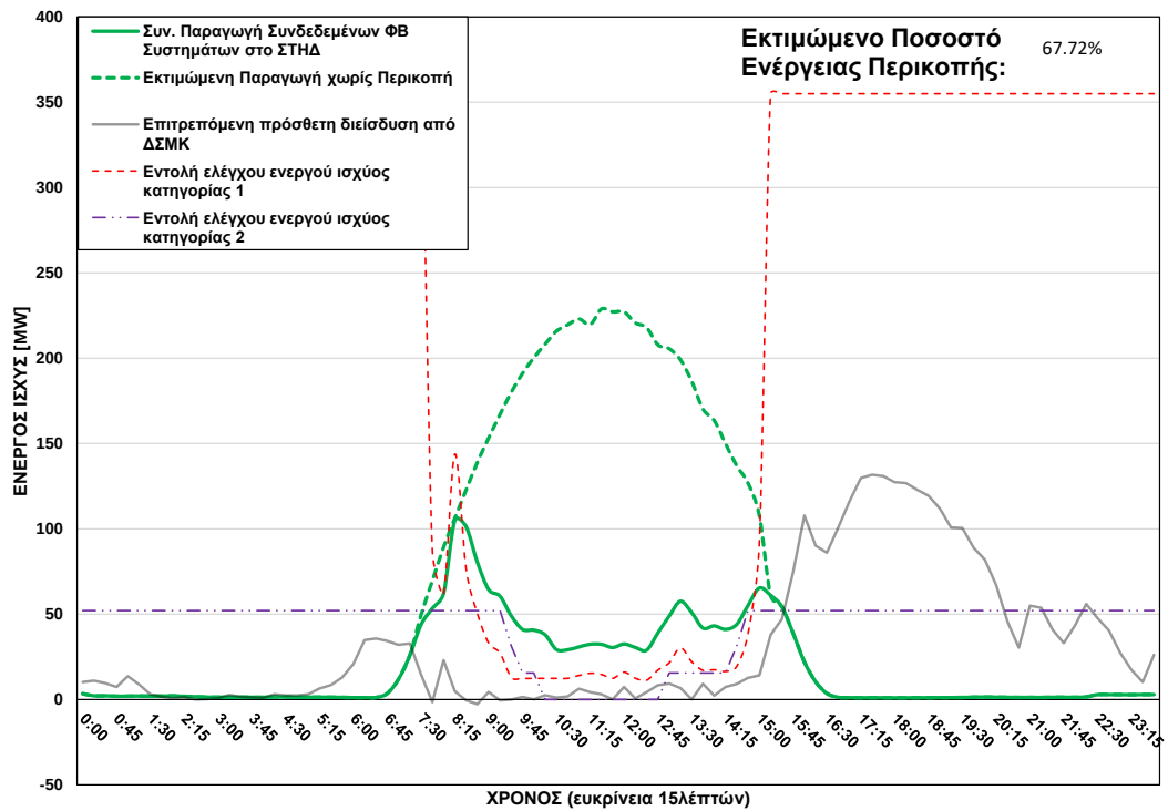
ΦΒ Παραγωγή στο ΣΤΗΔ στις 22/11/2025 (ώρα περικοπής: 07:30 - 15:00)
