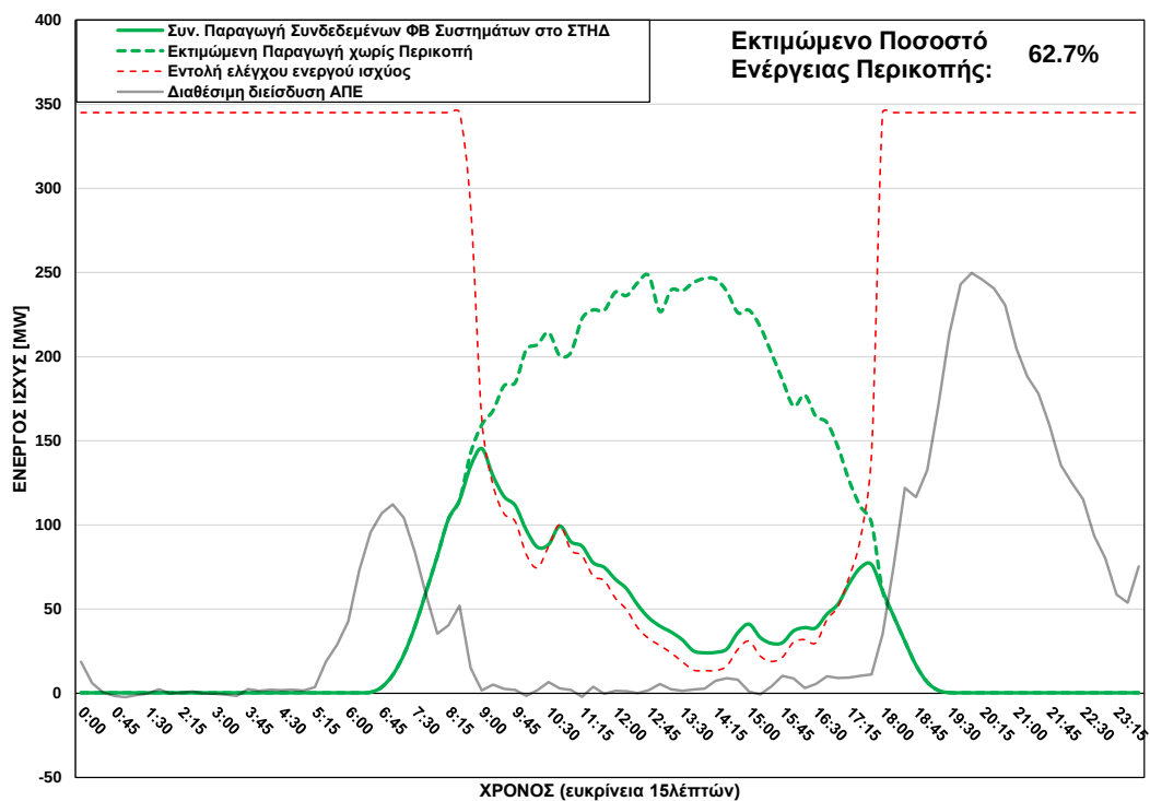
ΦΒ Παραγωγή στο ΣΤΗΔ στις 10/04/2025 (ώρα περικοπής: 08:45 - 17:45)
