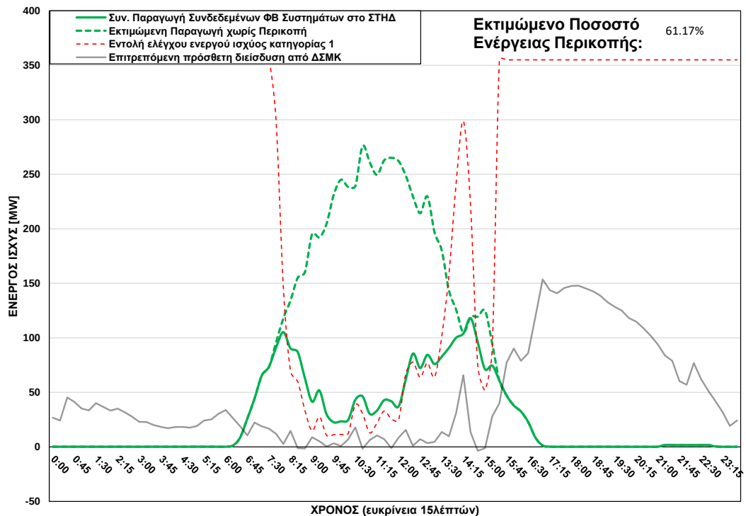
ΦΒ Παραγωγή στο ΣΤΗΔ στις 02/11/2025 (ώρα περικοπής: 07:45 - 15:15)
