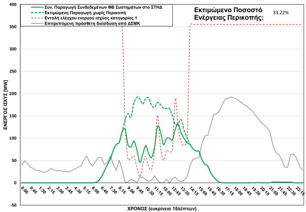
ΦΒ Παραγωγή στο ΣΤΗΔ στις 03/11/2025 (ώρα περικοπής: 08:45 - 14:00)
