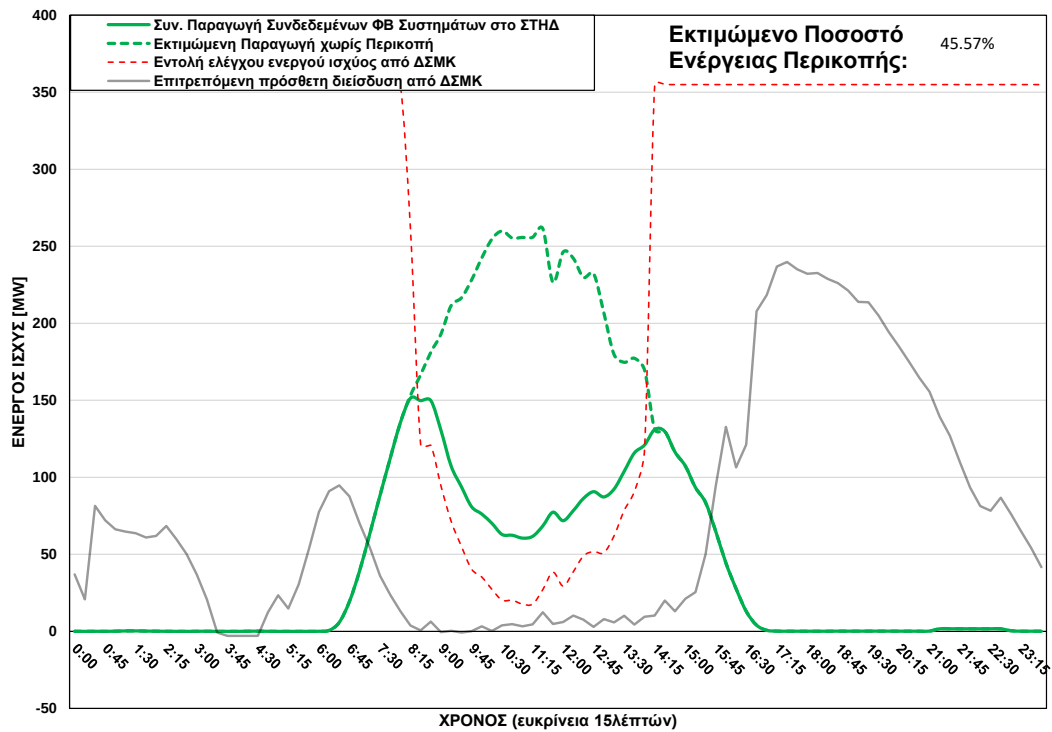
ΦΒ Παραγωγή στο ΣΤΗΔ στις 29/10/2025 (ώρα περικοπής: 08:15 - 14:00)
