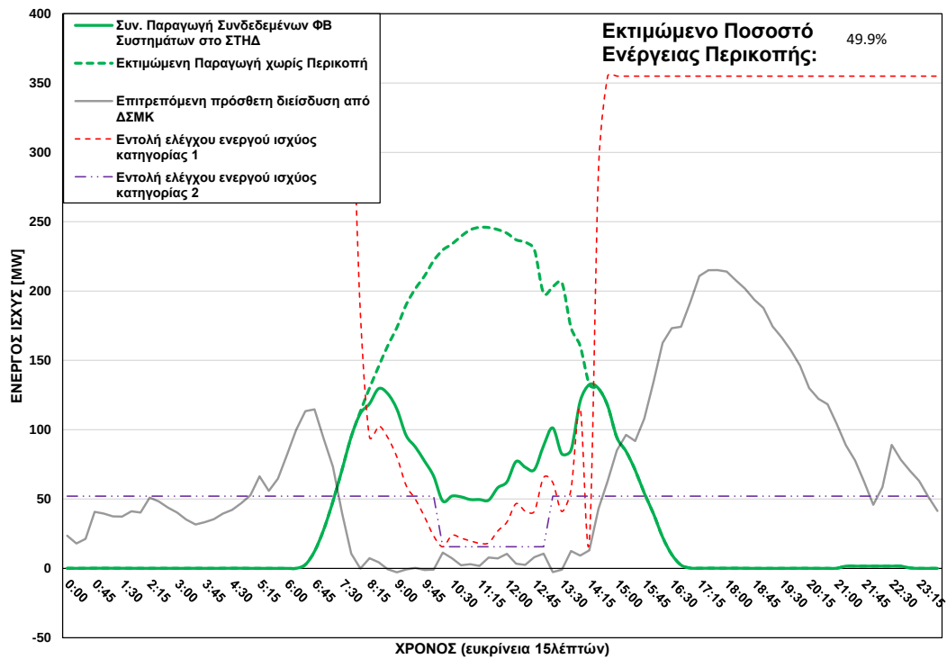
ΦΒ Παραγωγή στο ΣΤΗΔ στις 04/11/2025 (ώρα περικοπής: 08:00 - 14:00)
