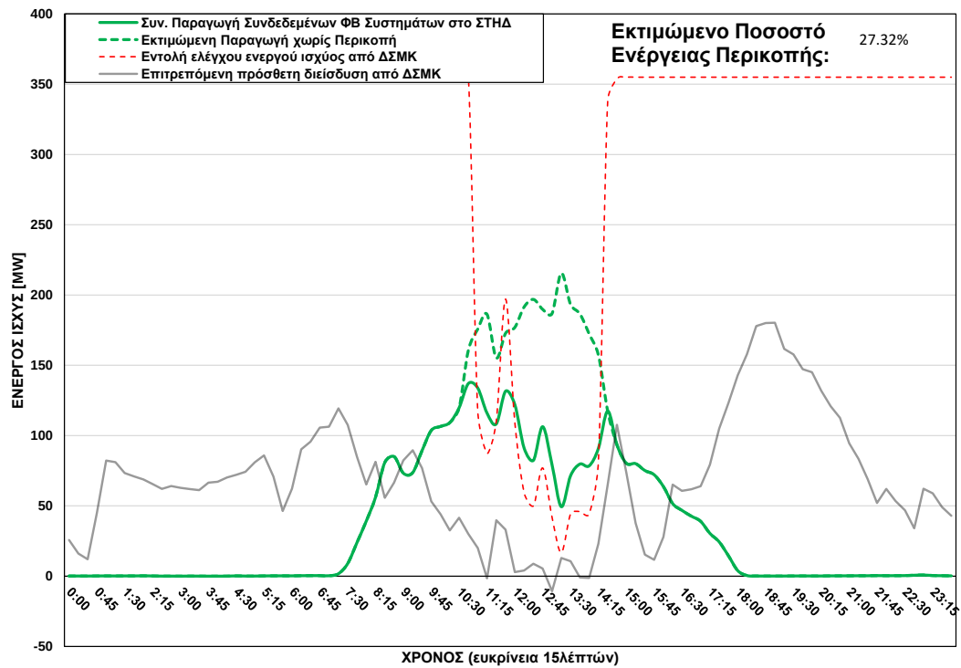
ΦΒ Παραγωγή στο ΣΤΗΔ στις 21/10/2025 (ώρα περικοπής: 10:45 - 14:15)
