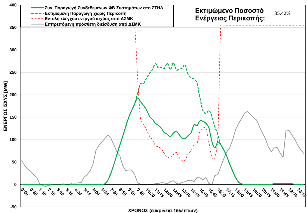
ΦΒ Παραγωγή στο ΣΤΗΔ στις 02/10/2025 (ώρα περικοπής: 09:45 - 16:30)
