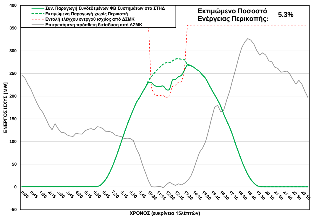
ΦΒ Παραγωγή στο ΣΤΗΔ στις 11/08/2025 (ώρα περικοπής: 10:30 - 13:30)
