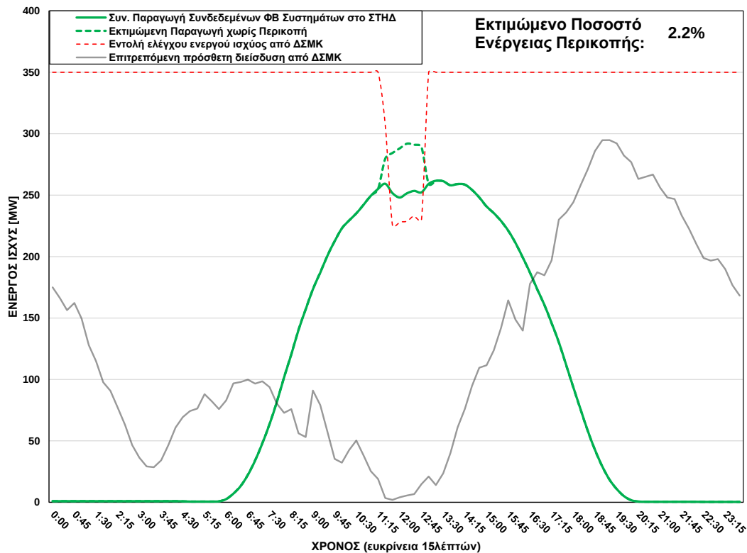
ΦΒ Παραγωγή στο ΣΤΗΔ στις 27/06/2025 (ώρα περικοπής: 11:30 - 12:45)
