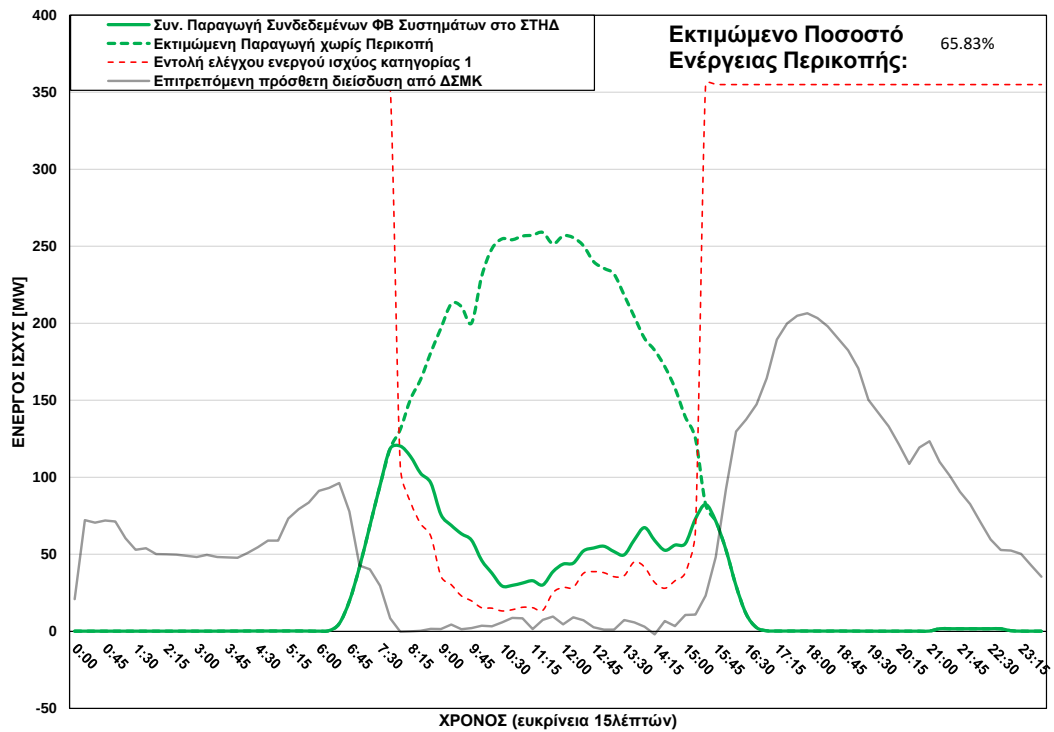
ΦΒ Παραγωγή στο ΣΤΗΔ στις 01/11/2025 (ώρα περικοπής: 08:00 - 15:15)
