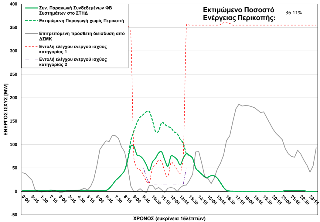
ΦΒ Παραγωγή στο ΣΤΗΔ στις 25/11/2025 (ώρα περικοπής: 08:45 - 13:00)
