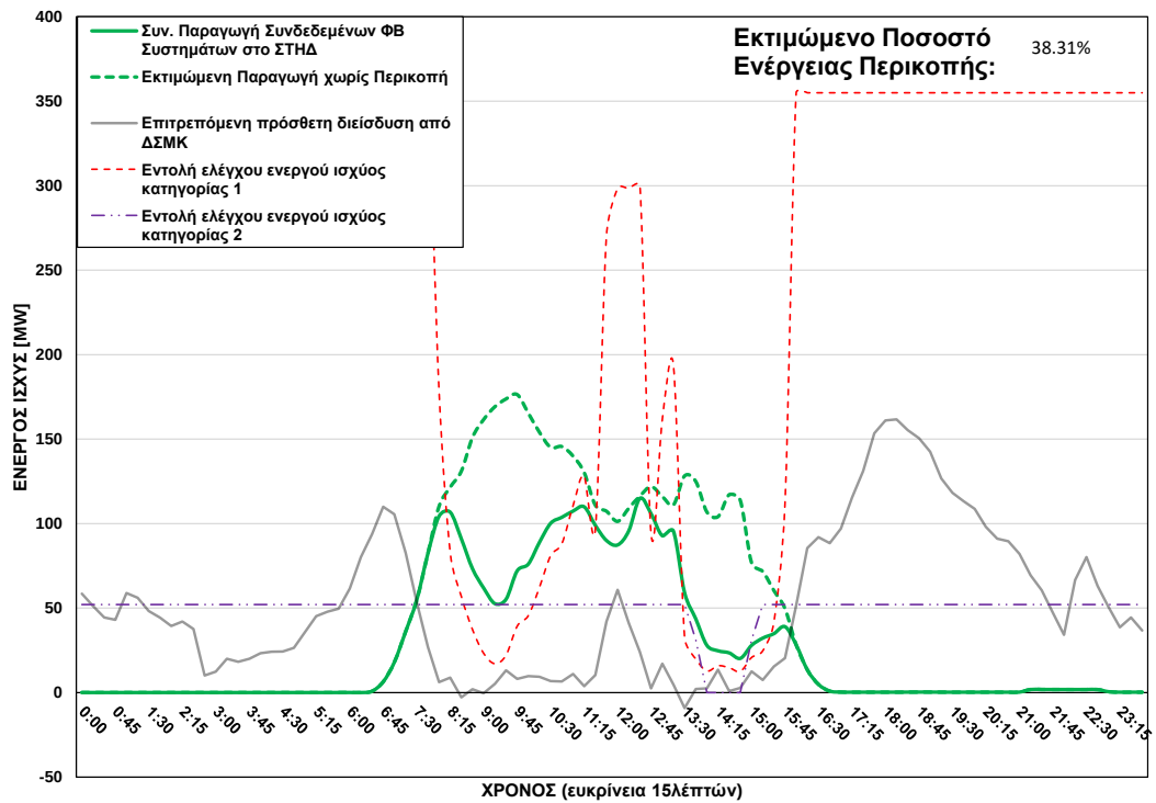
ΦΒ Παραγωγή στο ΣΤΗΔ στις 13/11/2025 (ώρα περικοπής: 08:00 - 15:45)
