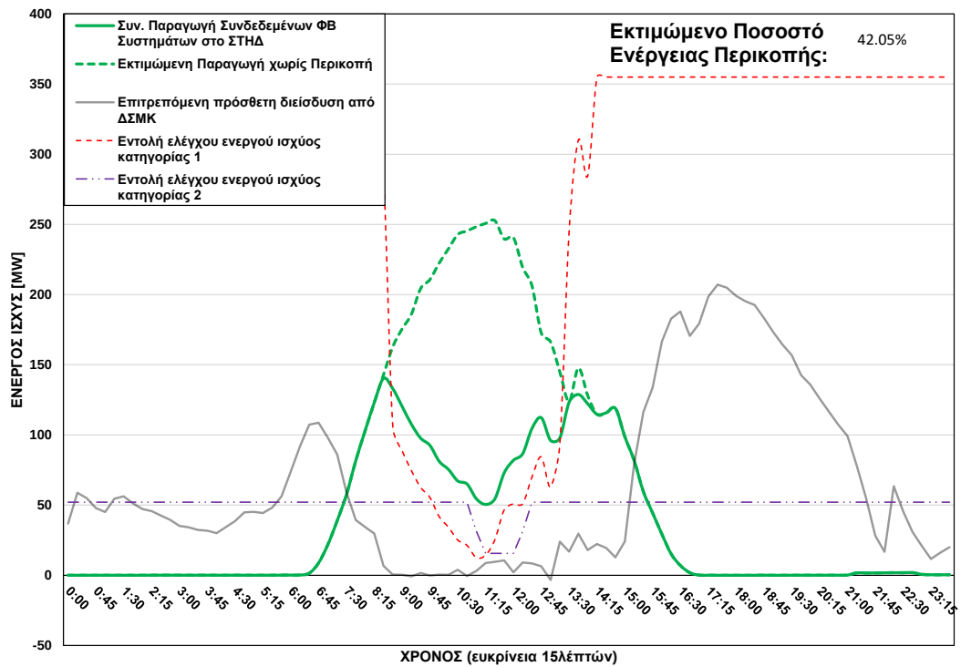
ΦΒ Παραγωγή στο ΣΤΗΔ στις 05/11/2025 (ώρα περικοπής: 08:30 - 14:00)
