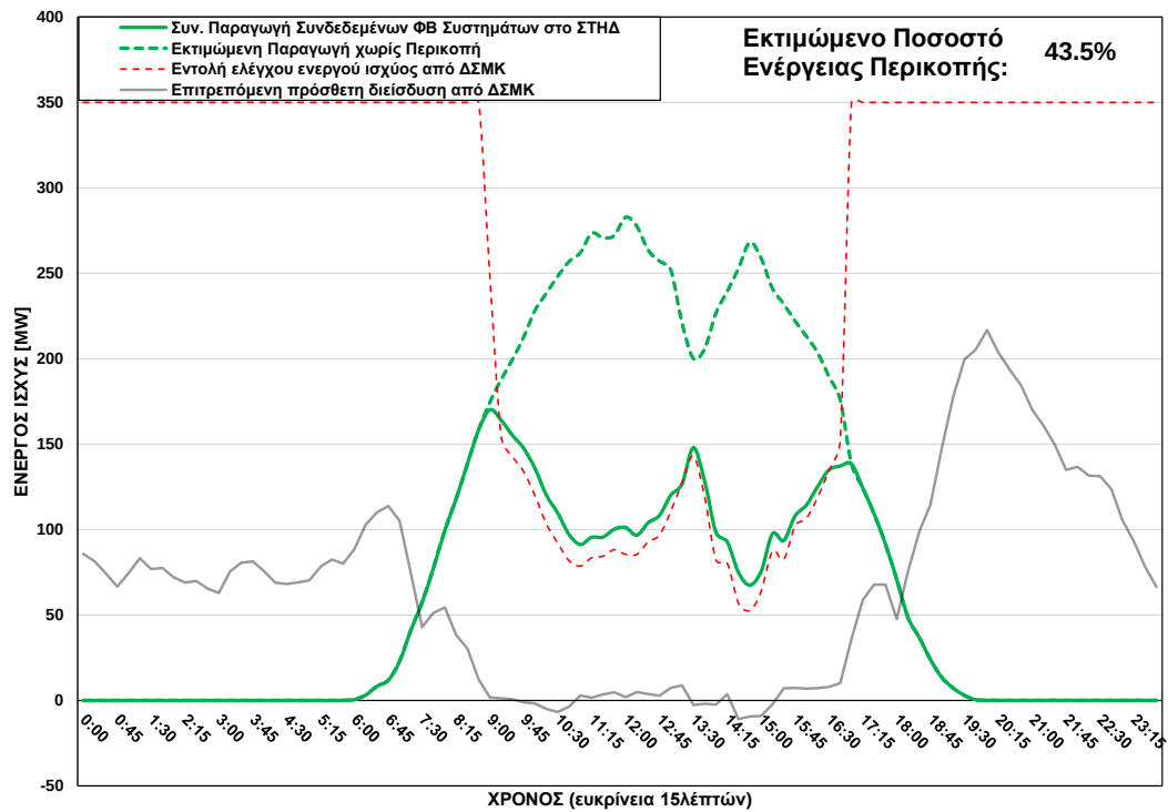
ΦΒ Παραγωγή στο ΣΤΗΔ στις 12/05/2025 (ώρα περικοπής: 09:00 - 16:45)
