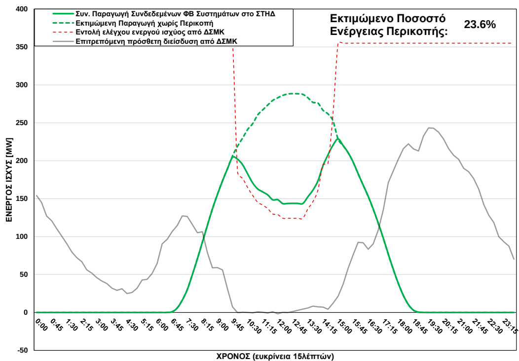
ΦΒ Παραγωγή στο ΣΤΗΔ στις 15/09/2025 (ώρα περικοπής: 09:45 - 14:45)
