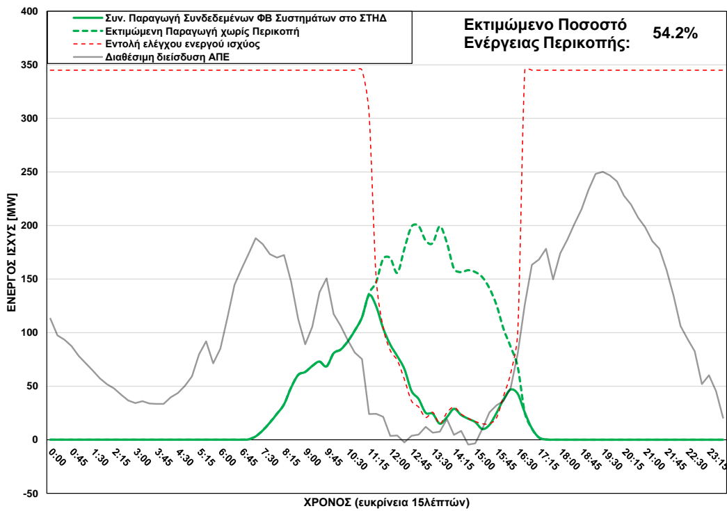
Φ/Β Παραγωγή στο ΣΤΗΔ στις 03/02/2025 (ώρα περικοπής: 11:15 - 16:30)
