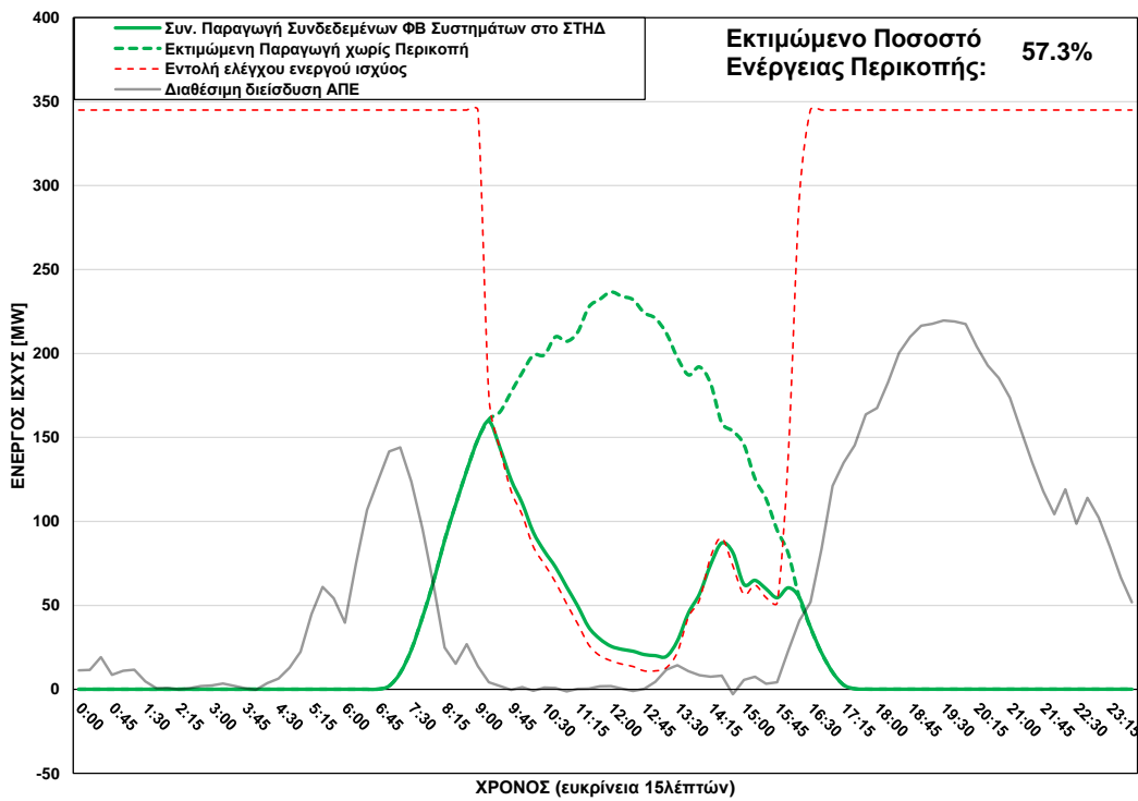
ΦΒ Παραγωγή στο ΣΤΗΔ στις 04/02/2025 (ώρα περικοπής: 09:15 - 16:00)
