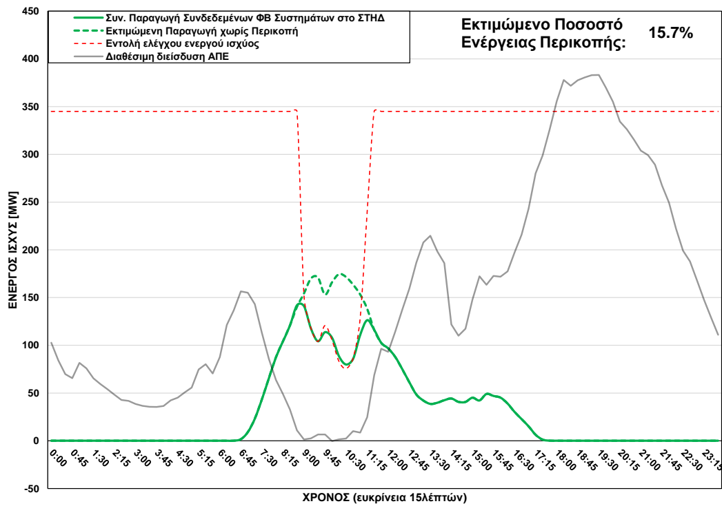
ΦΒ Παραγωγή στο ΣΤΗΔ στις 17/02/2025 (ώρα περικοπής: 08:45 - 11:15)
