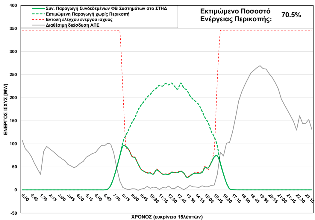
Φ/Β Παραγωγή στο ΣΤΗΔ στις 02/02/2025 (ώρα περικοπής: 08:15 - 16:00)
