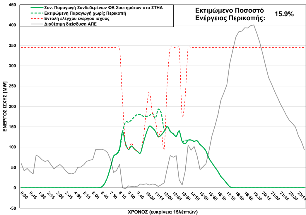
ΦΒ Παραγωγή στο ΣΤΗΔ στις 22/02/2025 (ώρα περικοπής: 08:15 - 13:45)
