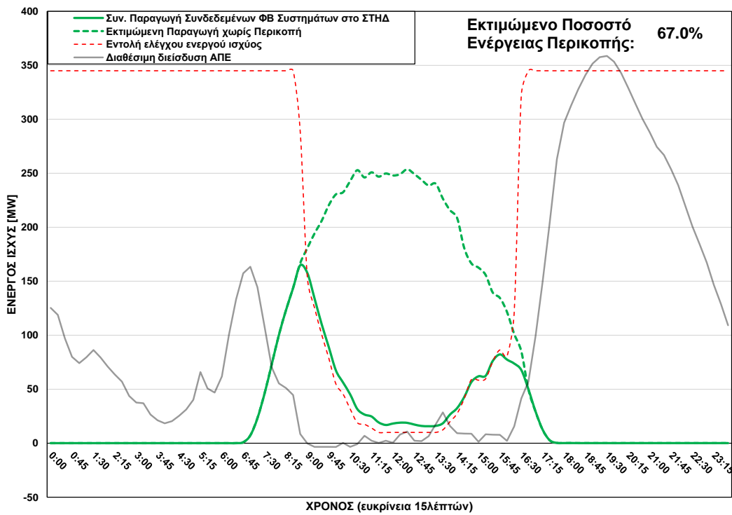
Φ/Β Παραγωγή στο ΣΤΗΔ στις 14/02/2025 (ώρα περικοπής: 08:45 - 16:30)
