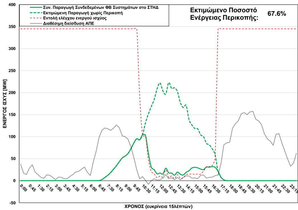
Φ/Β Παραγωγή στο ΣΤΗΔ στις 19/02/2025 (ώρα περικοπής: 10:45 - 16:45)
