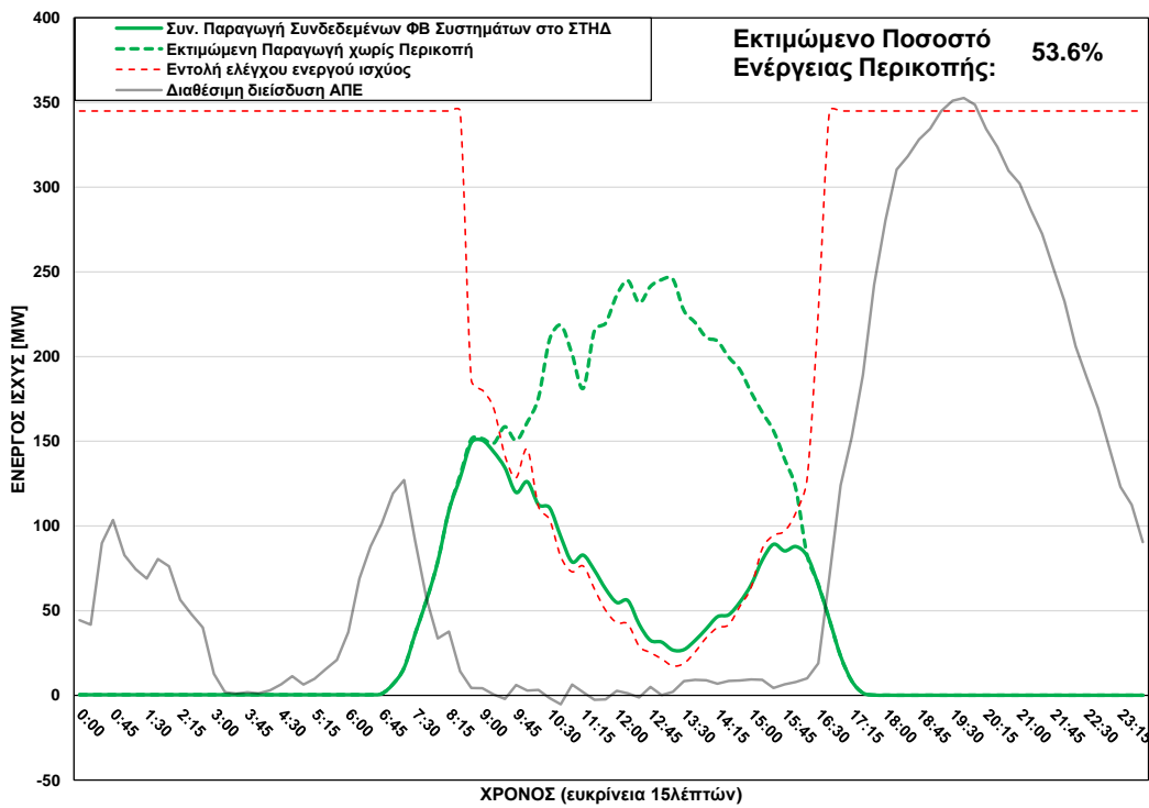
Φ/Β Παραγωγή στο ΣΤΗΔ στις 13/02/2025 (ώρα περικοπής: 08:30 - 16:00)
