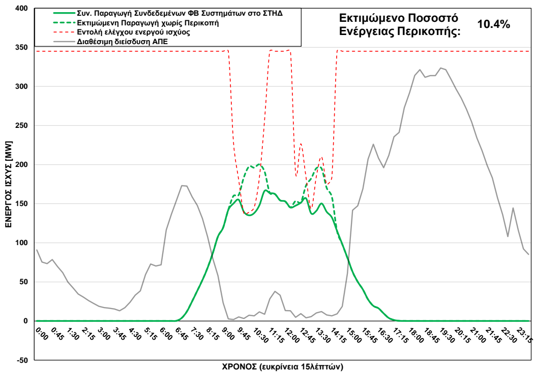
ΦΒ Παραγωγή στο ΣΤΗΔ στις 10/02/2025 (ώρα περικοπής: 09:30 - 14:15)
