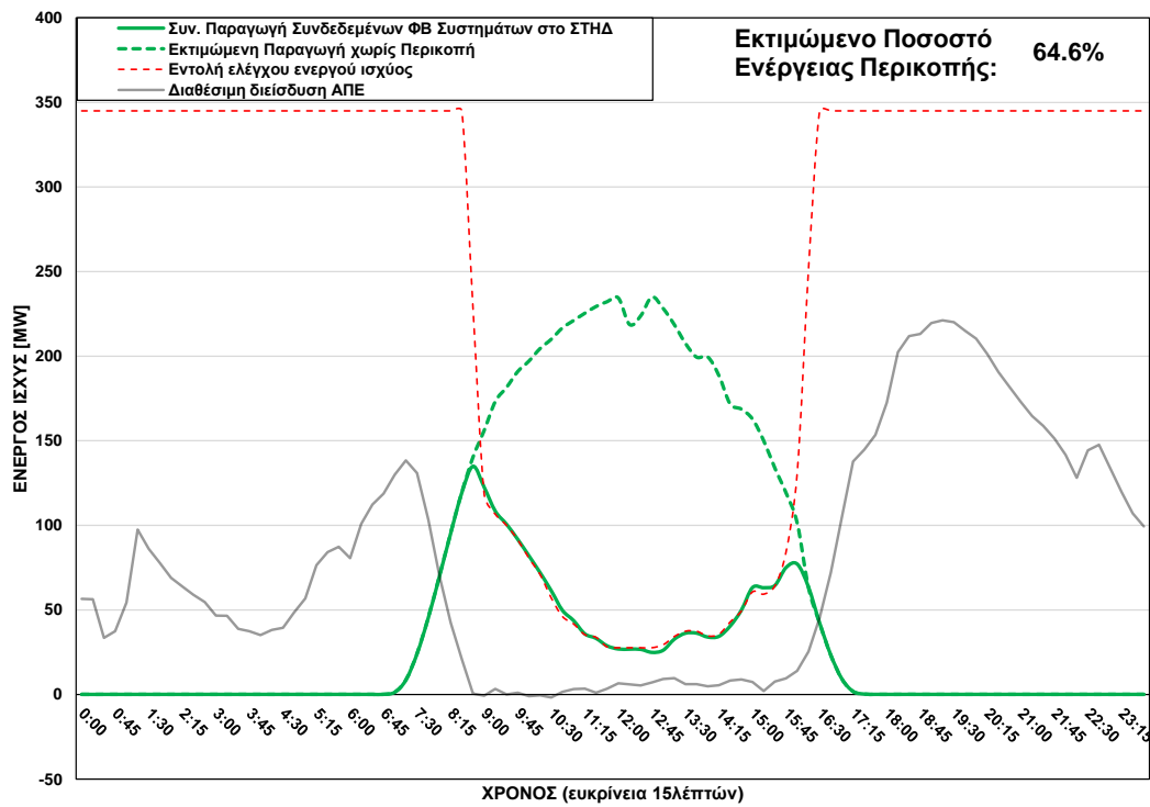
Φ/Β Παραγωγή στο ΣΤΗΔ στις 01/02/2025 (ώρα περικοπής: 08:45 - 16:00)
