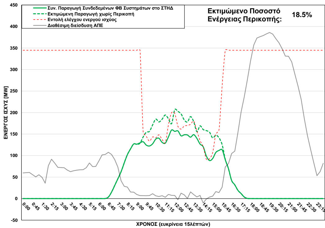
ΦΒ Παραγωγή στο ΣΤΗΔ στις 23/02/2025 (ώρα περικοπής: 09:30 - 15:45)
