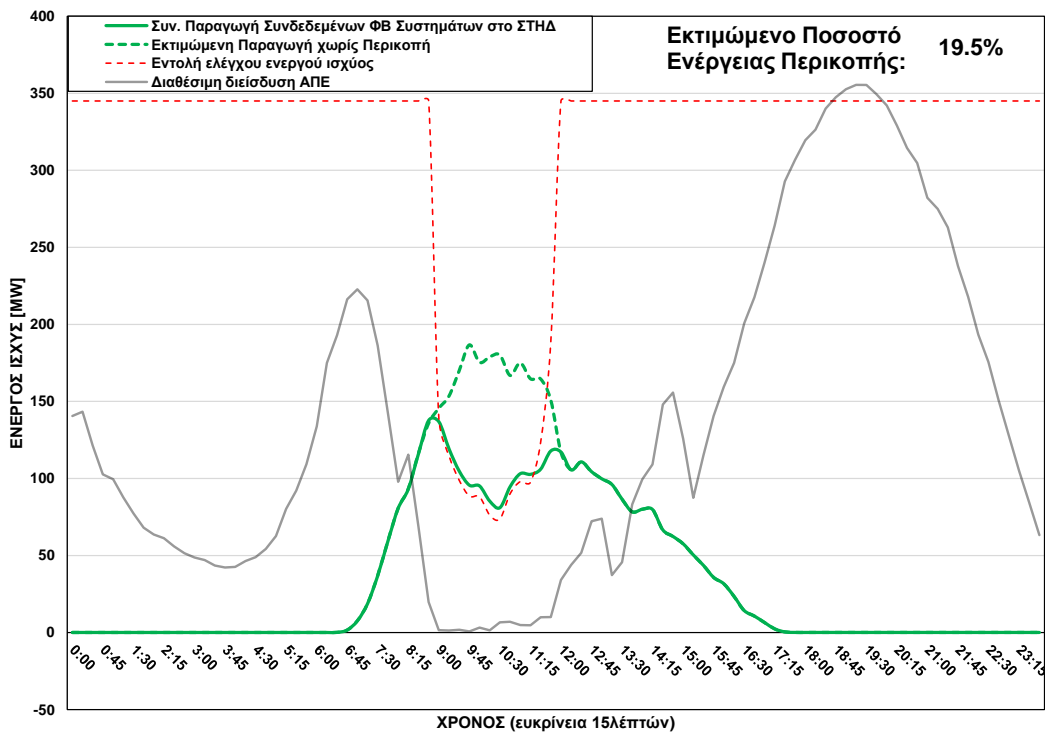
ΦΒ Παραγωγή στο ΣΤΗΔ στις 18/02/2025 (ώρα περικοπής: 08:45 - 11:45)
