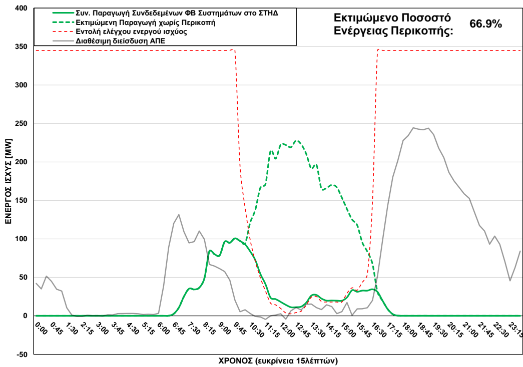
Φ/Β Παραγωγή στο ΣΤΗΔ στις 20/02/2025 (ώρα περικοπής: 10:15 - 16:30)
