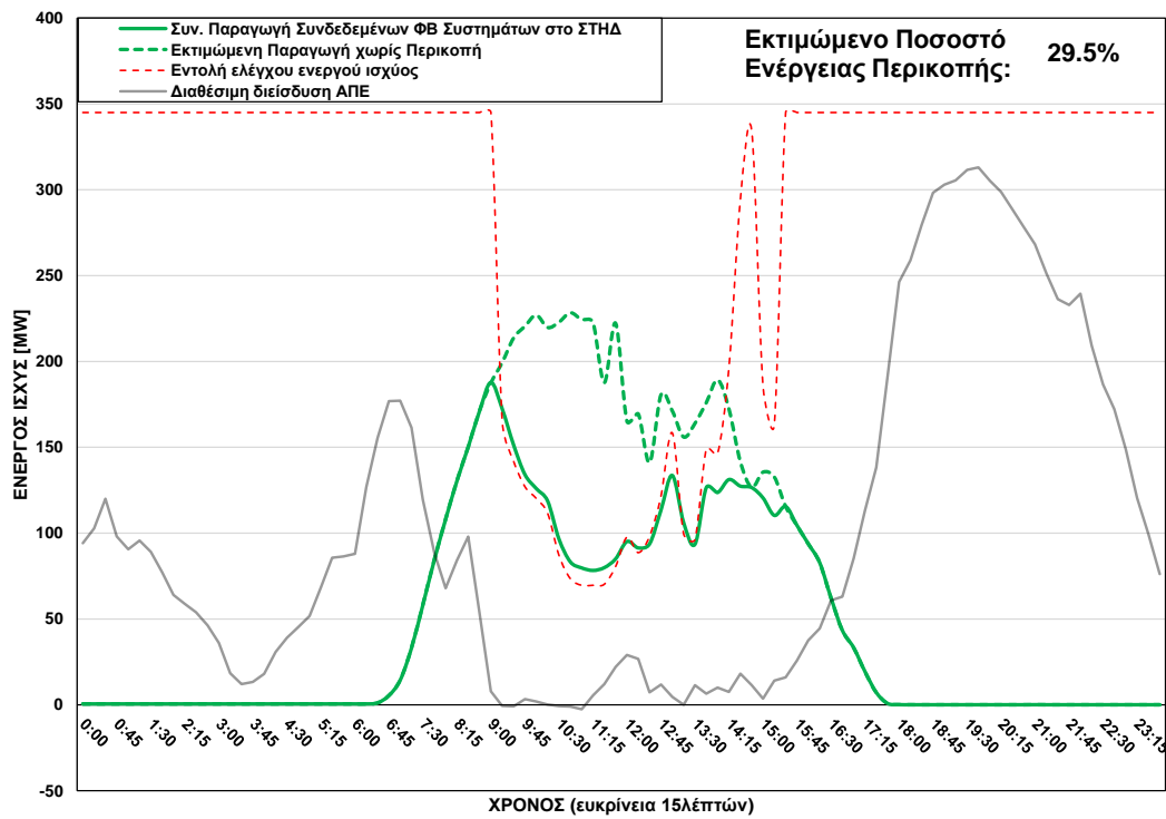
ΦΒ Παραγωγή στο ΣΤΗΔ στις 27/02/2025 (ώρα περικοπής: 09:15 - 15:15)
