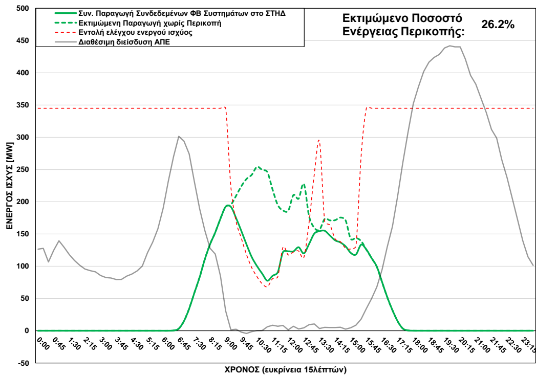
ΦΒ Παραγωγή στο ΣΤΗΔ στις 25/02/2025 (ώρα περικοπής: 09:15 - 15:30)
