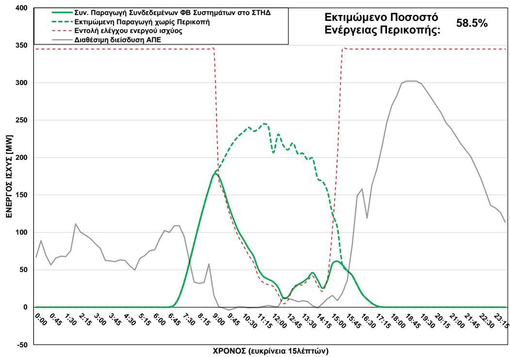
ΦΒ Παραγωγή στο ΣΤΗΔ στις 08/02/2025 (ώρα περικοπής: 09:15 - 15:15)
