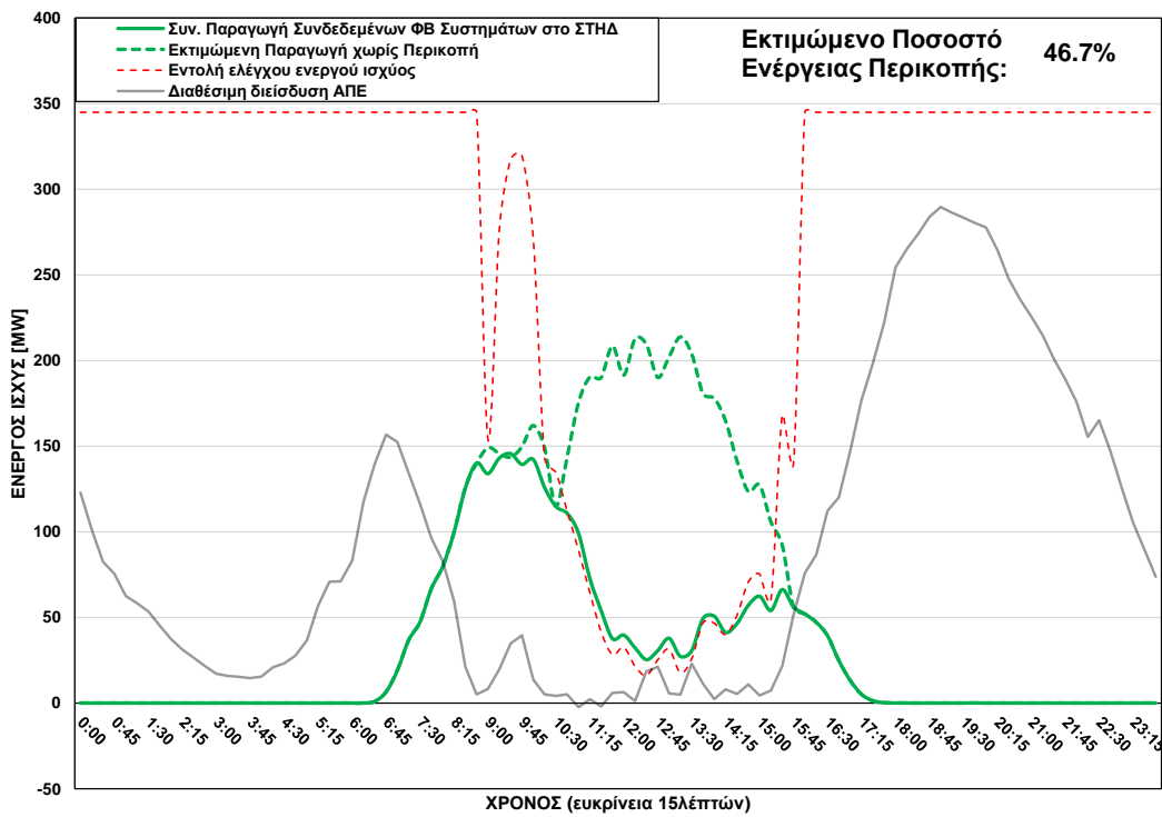
Φ/Β Παραγωγή στο ΣΤΗΔ στις 28/02/2025 (ώρα περικοπής: 09:00 - 15:30)
