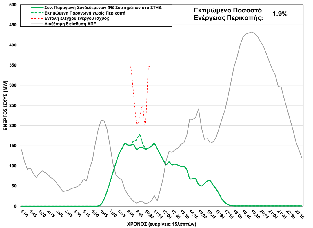
ΦΒ Παραγωγή στο ΣΤΗΔ στις 26/02/2025 (ώρα περικοπής: 09:30 - 10:30)
