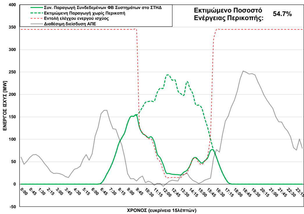
Φ/Β Παραγωγή στο ΣΤΗΔ στις 21/02/2025 (ώρα περικοπής: 10:00 - 16:00)
