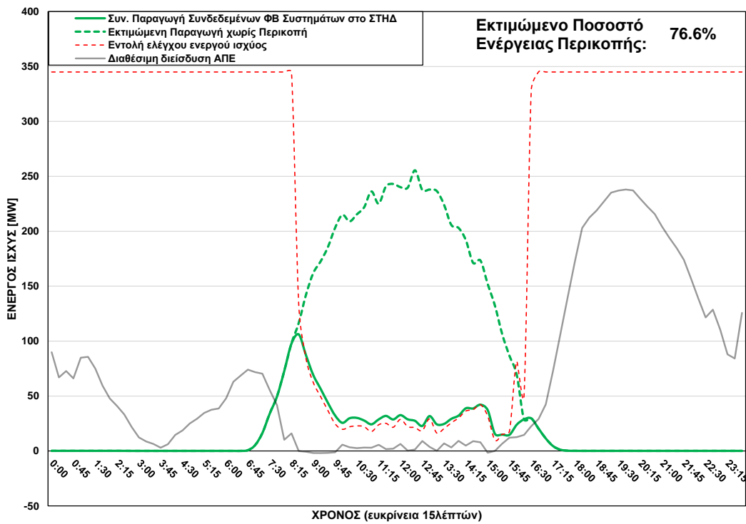
Φ/Β Παραγωγή στο ΣΤΗΔ στις 16/02/2025 (ώρα περικοπής: 08:30 - 16:00)
