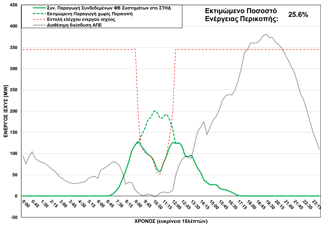
ΦΒ Παραγωγή στο ΣΤΗΔ στις 09/02/2025 (ώρα περικοπής: 09:15 - 12:00)
