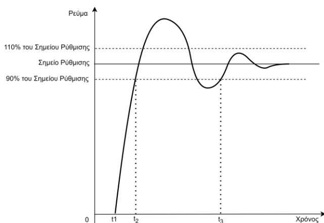
Σχεδιάγραμμα Δ5.6: Χρόνος Ανταπόκρισης ρύθμισης Ταχύς Ρεύματος Σφάλματος
