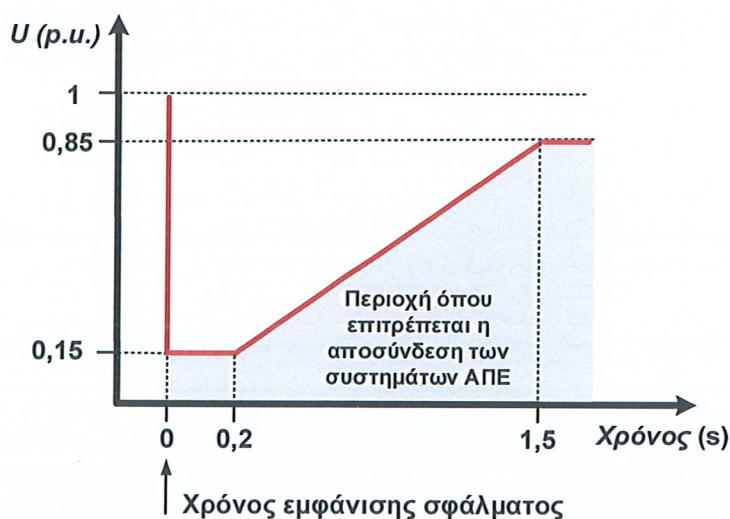
ΣΧΕΔΙΑΓΡΑΜΜΑ 1: Χαρακτηριστική καμπύλη UVRT
